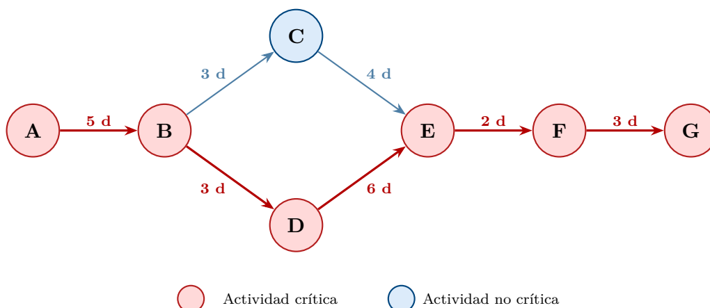
Figura 2: Diagrama de red PERT/CPM. Rojo: ruta crítica A \rightarrow B \rightarrow D \rightarrow E \rightarrow F \rightarrow G .
