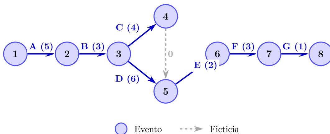
Figura 2: Diagrama de red AOA.
