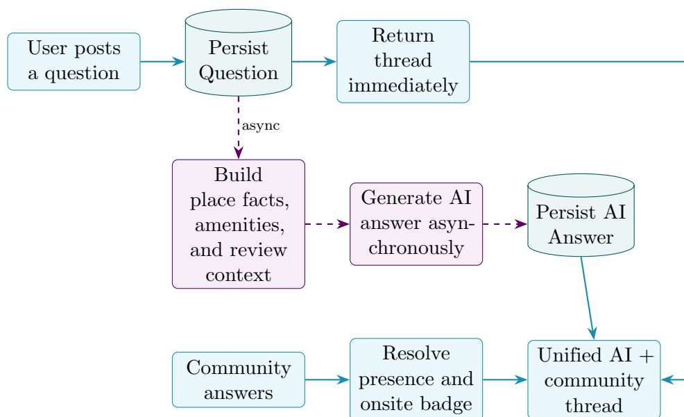
Hình 16: Luồng Hỏi - Đáp bất đồng bộ kết hợp câu trả lời từ AI với kiến thức của cộng đồng tại chỗ.
