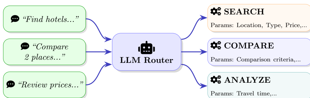
Hình 1: Mẫu truy vấn — Chuẩn hóa các truy vấn tự nhiên đa dạng thành tham số điều hướng.
