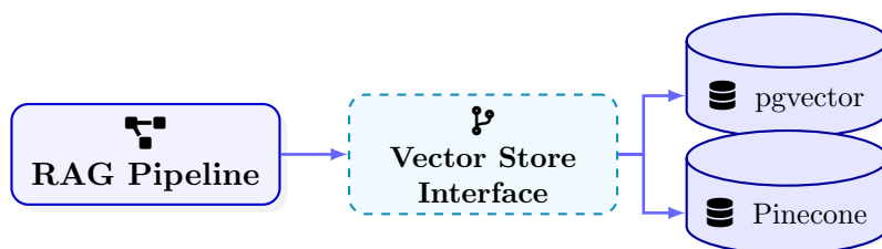
Hình 9: Trừu tượng hóa Lưu trữ Vector
