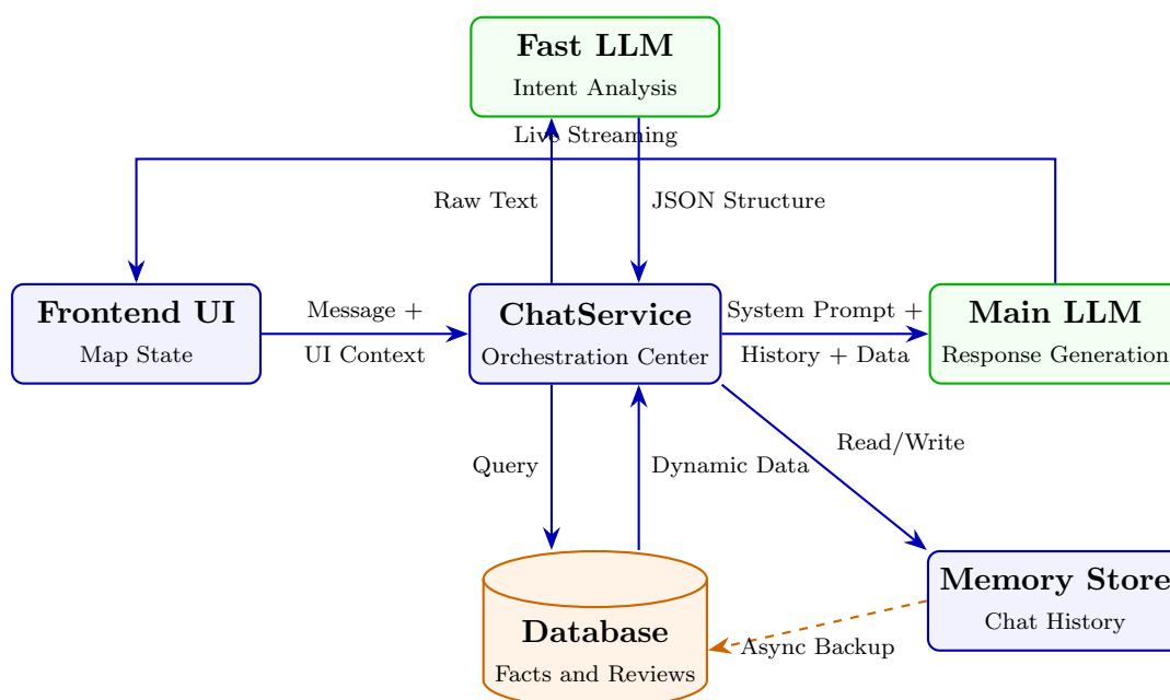
Hình 19: Luồng Quản lý Context LLM — Minh họa luồng dữ liệu quản lý ngữ cảnh từ giao diện người dùng (UI) đến LLM.
