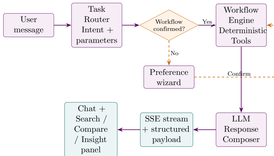
Hình 15: Luồng điều phối AI sử dụng mô hình Router–Confirmation–Engine–Composer.
