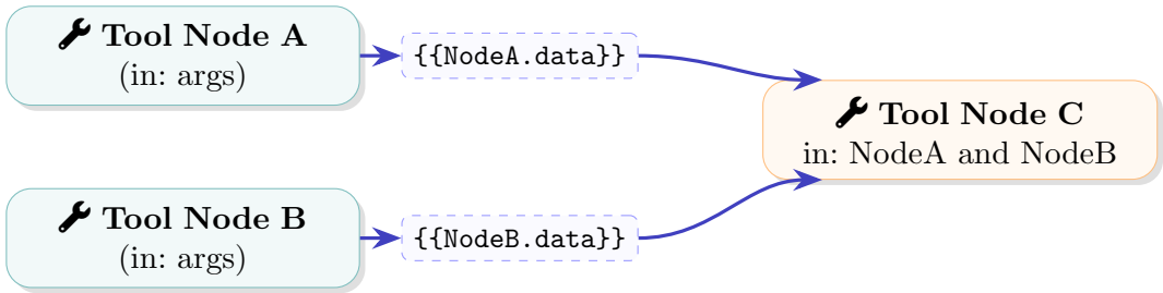
Hình 6: Mẫu công cụ Workflow — Nhận diện các mẫu phụ thuộc dữ liệu bằng cách sử dụng Chuỗi mẫu (String Templates) giữa các Công cụ.
