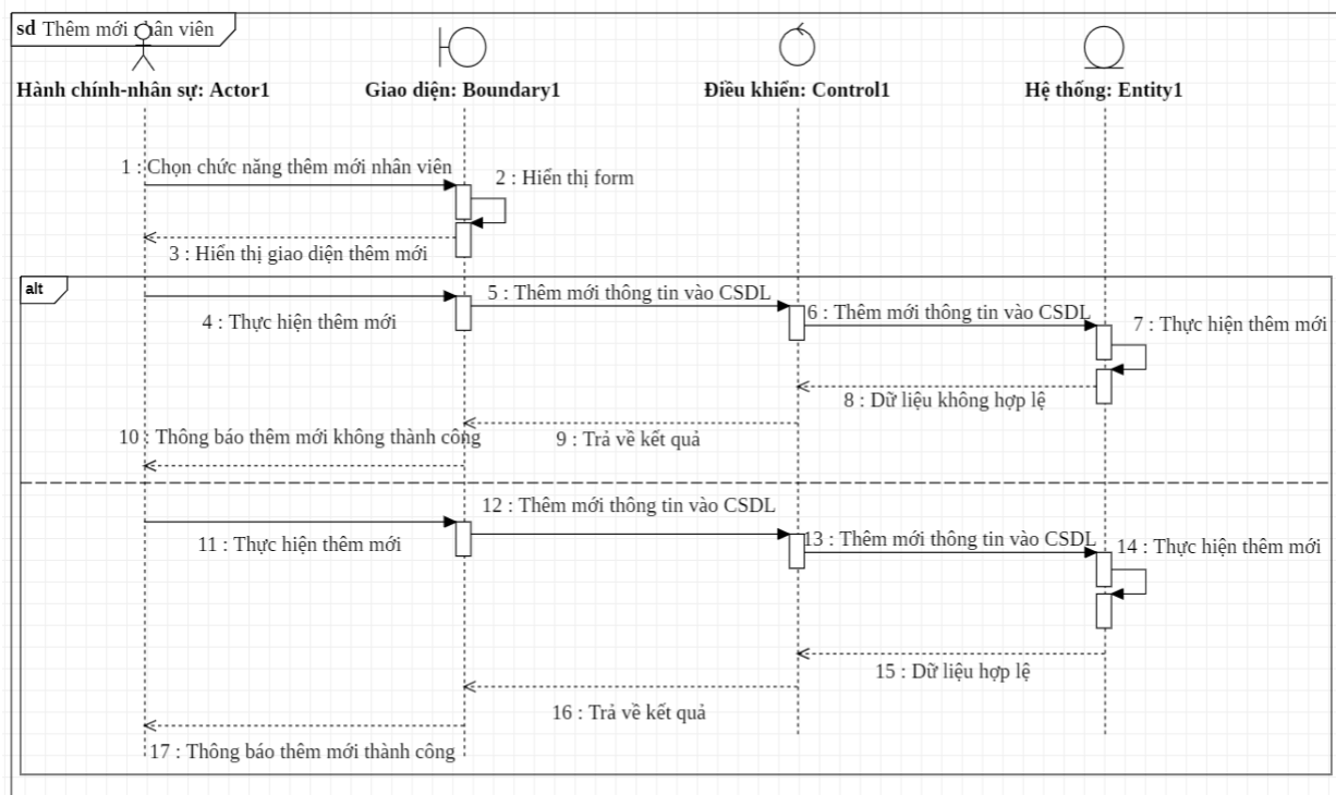
Hình 2.8: Biểu đồ tuần tự thêm mới nhân viên
