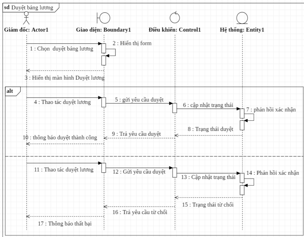
Hình 2.10: Biểu đồ giám đốc duyệt bảng lương
