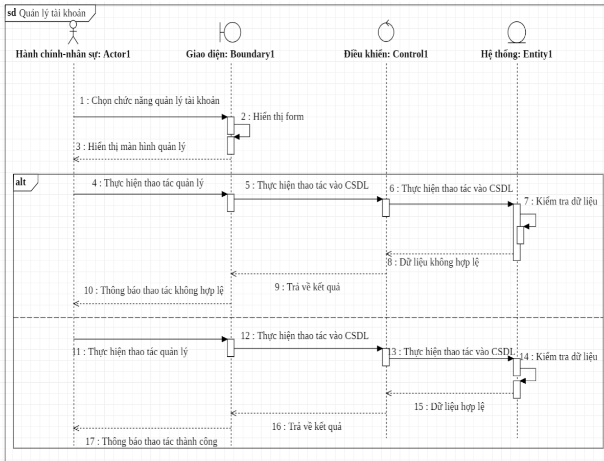
Hình 2.9: Biểu đồ quản lý tài khoản
