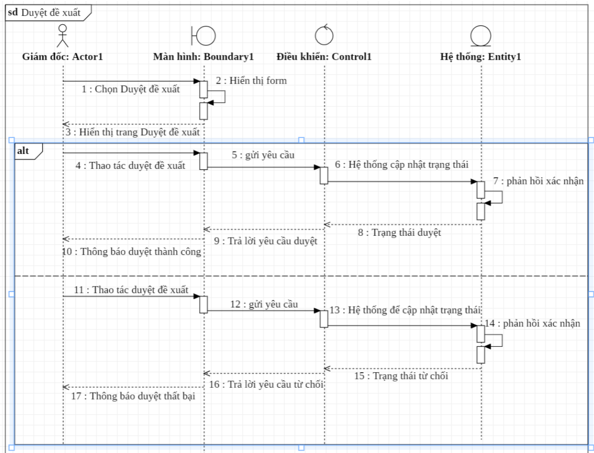
Hình 2.11 Biểu đồ giám đốc duyệt đề xuất
