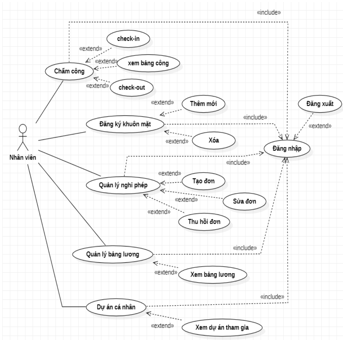
Hình 2.2 Biểu đồ Use Case phân rã theo tác nhân – Nhân viên
