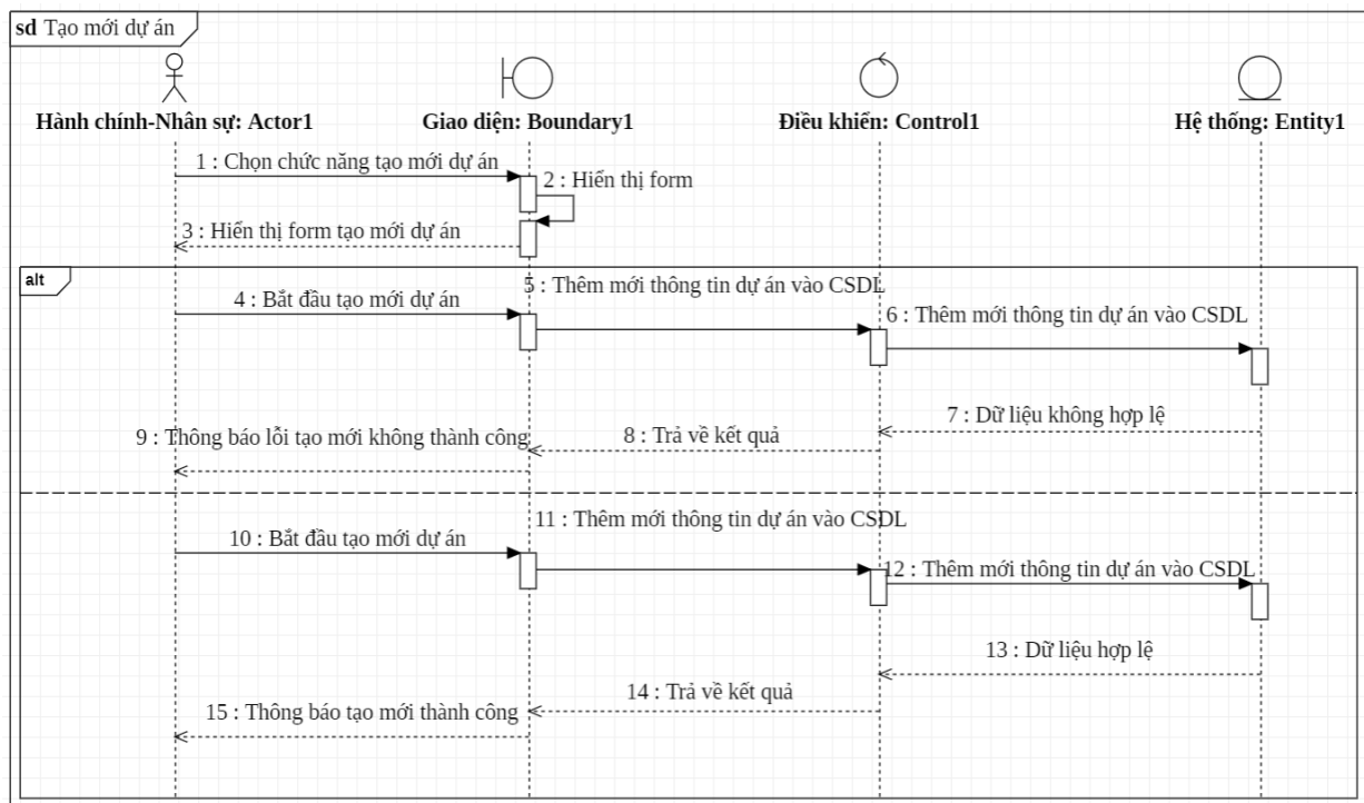
Hình 2.7: Biểu đồ tuần tự tạo mới dự án
