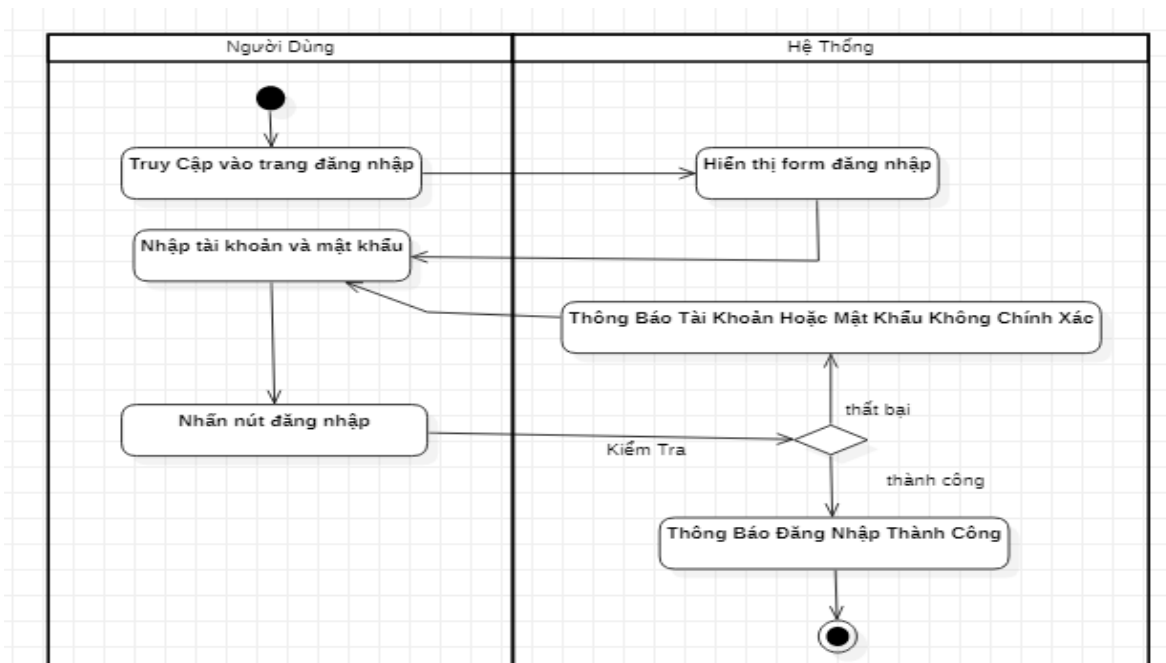
Hình 2.13 Biểu đồ hoạt động đăng nhập
