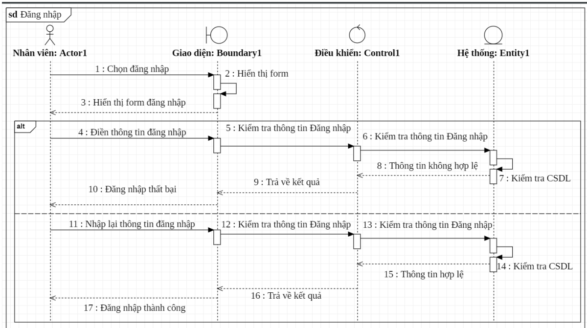
Hình 2.5: Biểu đồ tuần tự chức năng đăng nhập
