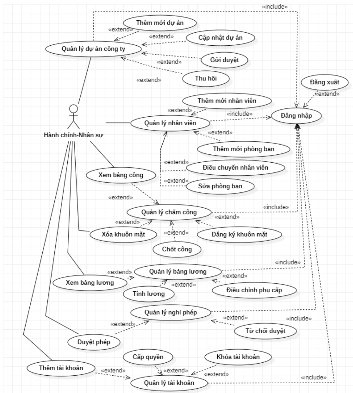
Hình 2.3 Biểu đồ Use Case phân rã theo tác nhân – Hành chính-Nhân sự
