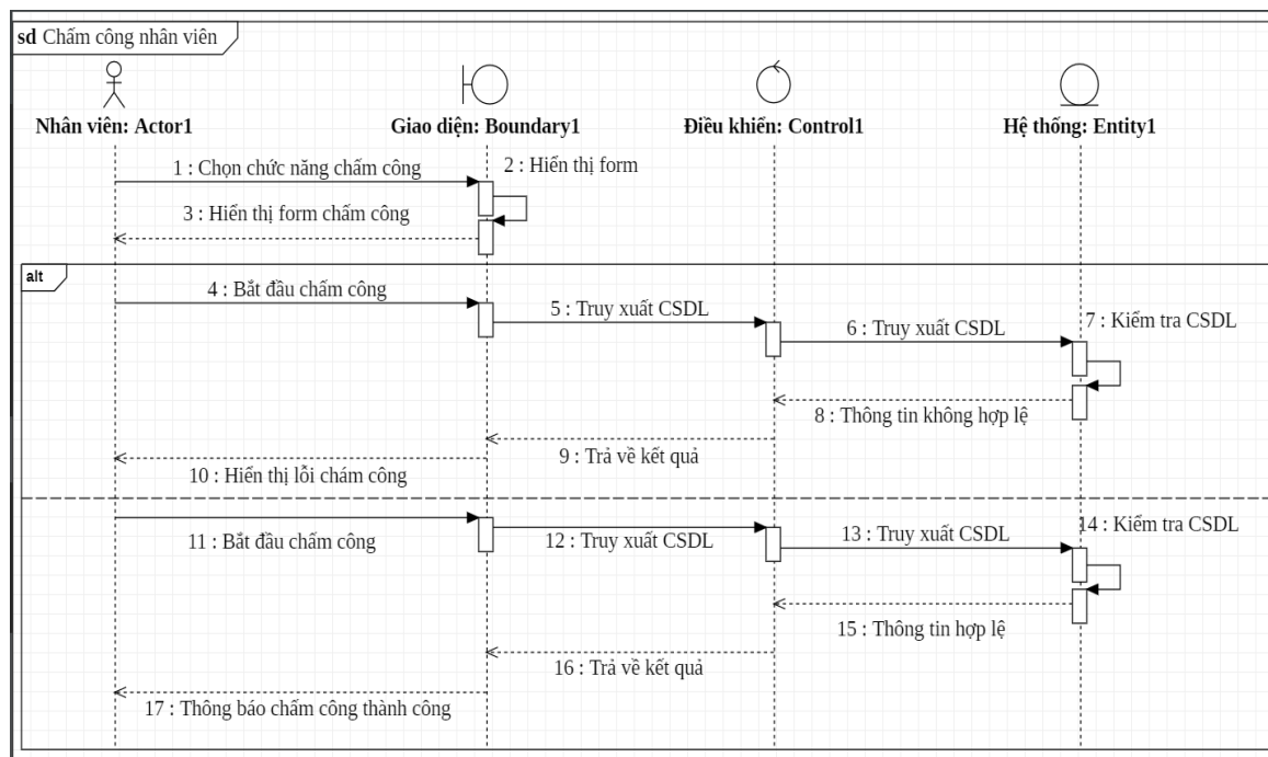
Hình 2.6: Biểu đồ tuần tự chức năng chấm công Nhân viên
