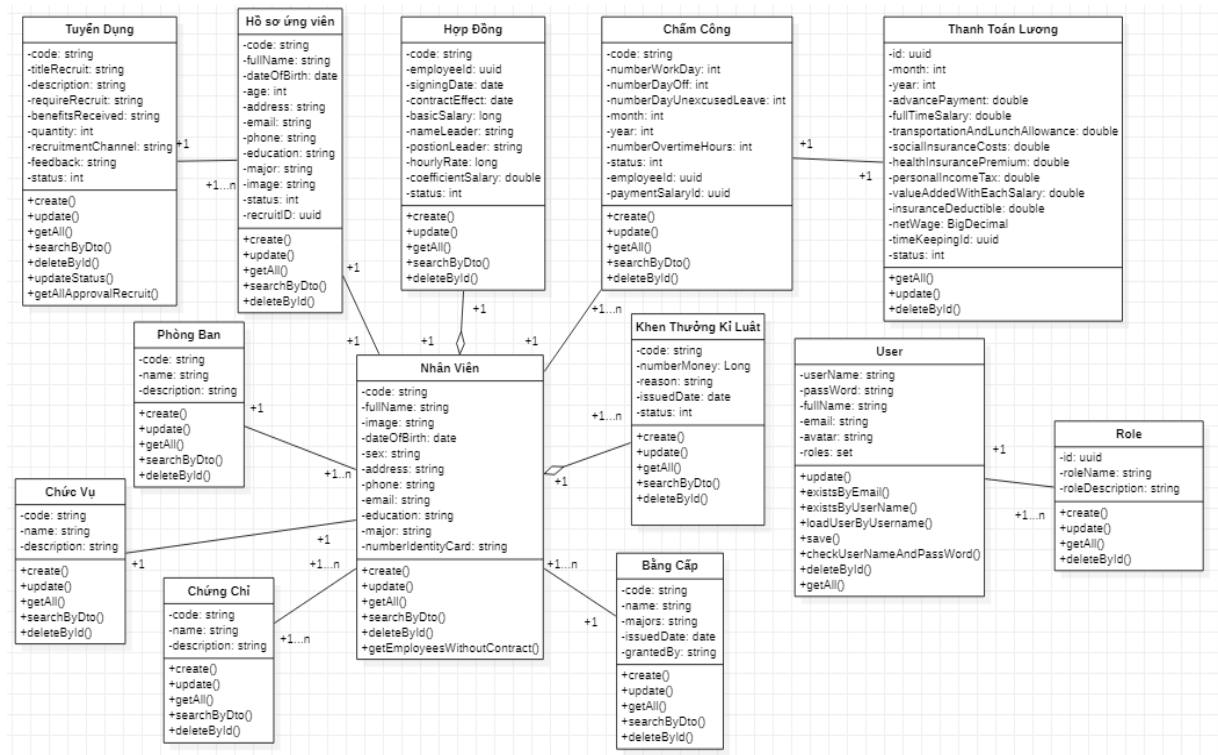
Hình 2.12 Biểu đồ lớp chi tiết
