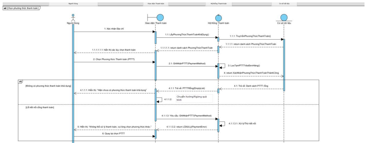
Hình 5.1.8.3. Sequence Diagram Chọn phương thức thanh toán
