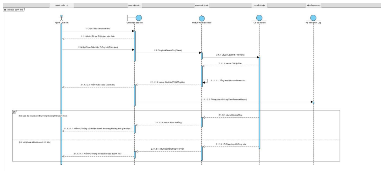
Hình 5.2.6.4. Sequence Diagram Báo cáo doanh thu
