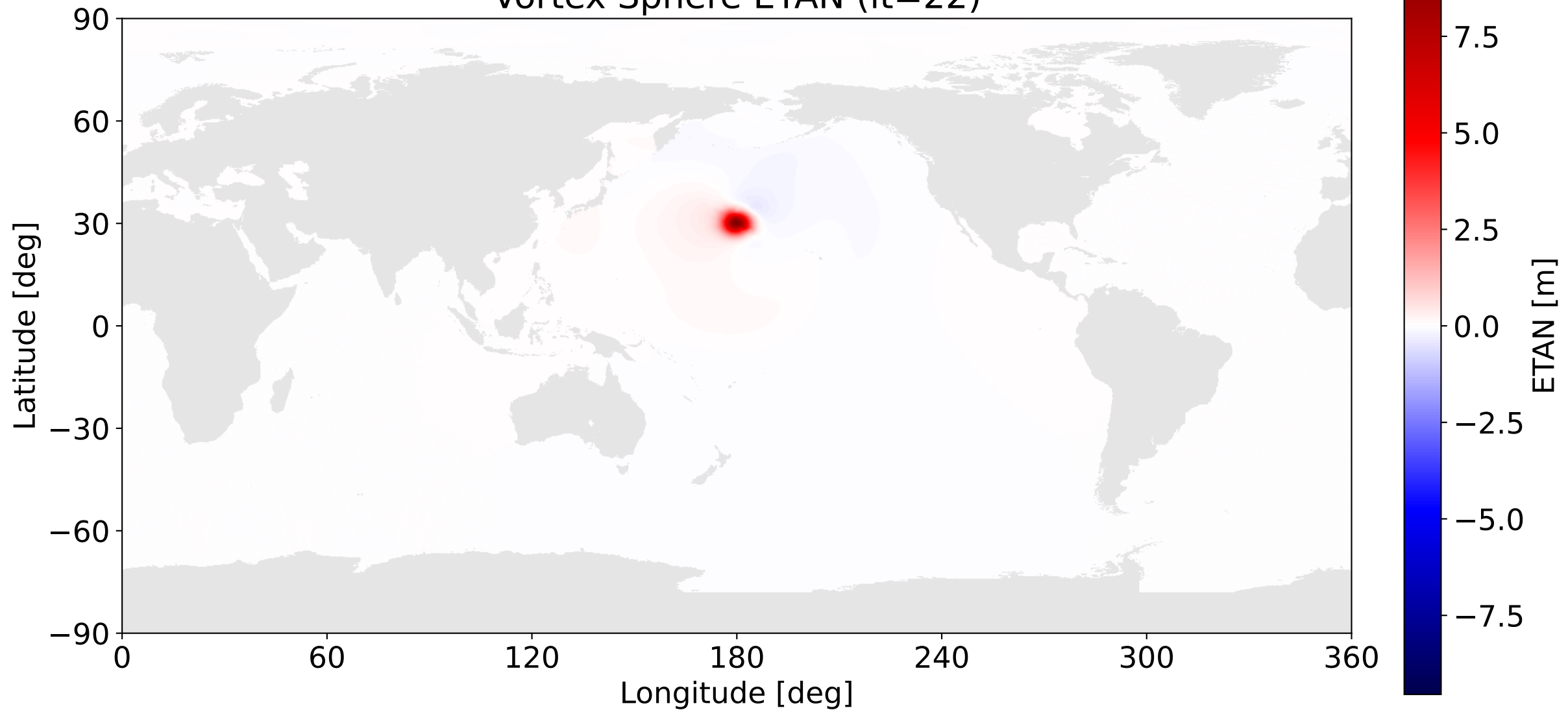
Vortex Sphere ETAN (it=22)
