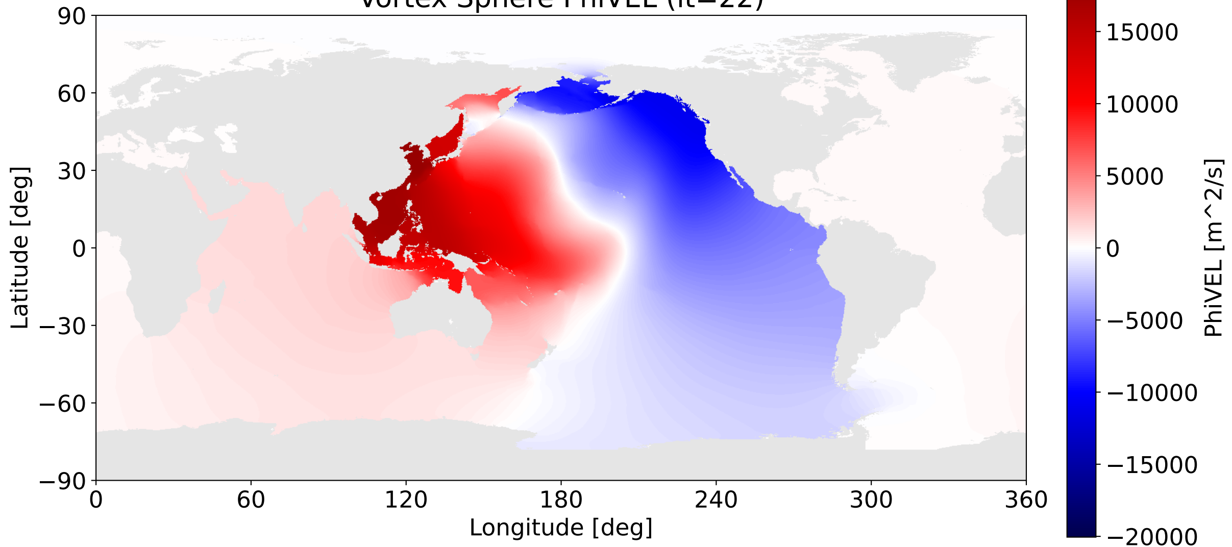
Vortex Sphere PhiVEL (it=22)
