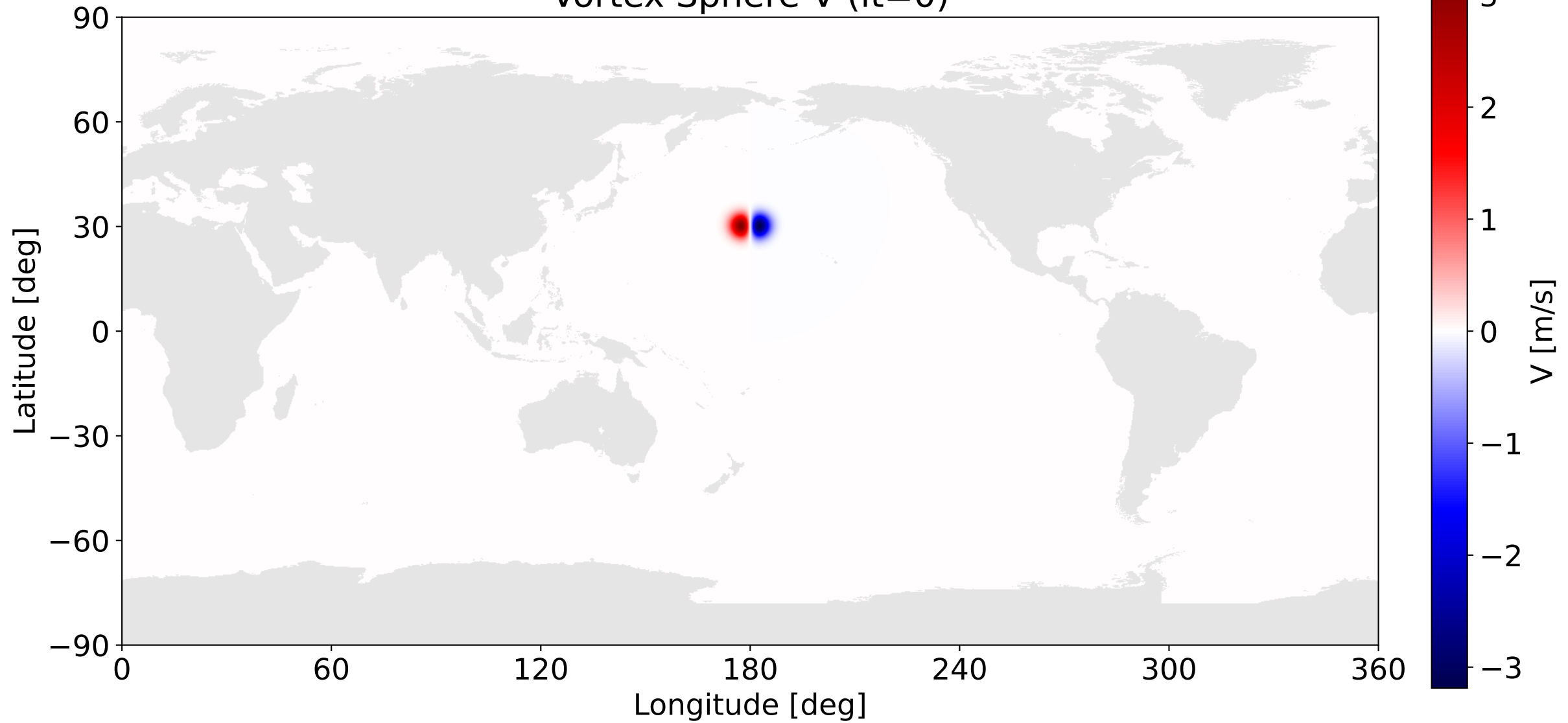
Vortex Sphere V (it=0)
