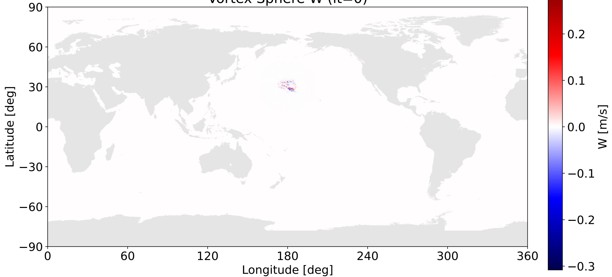
Vortex Sphere W (it=0)
