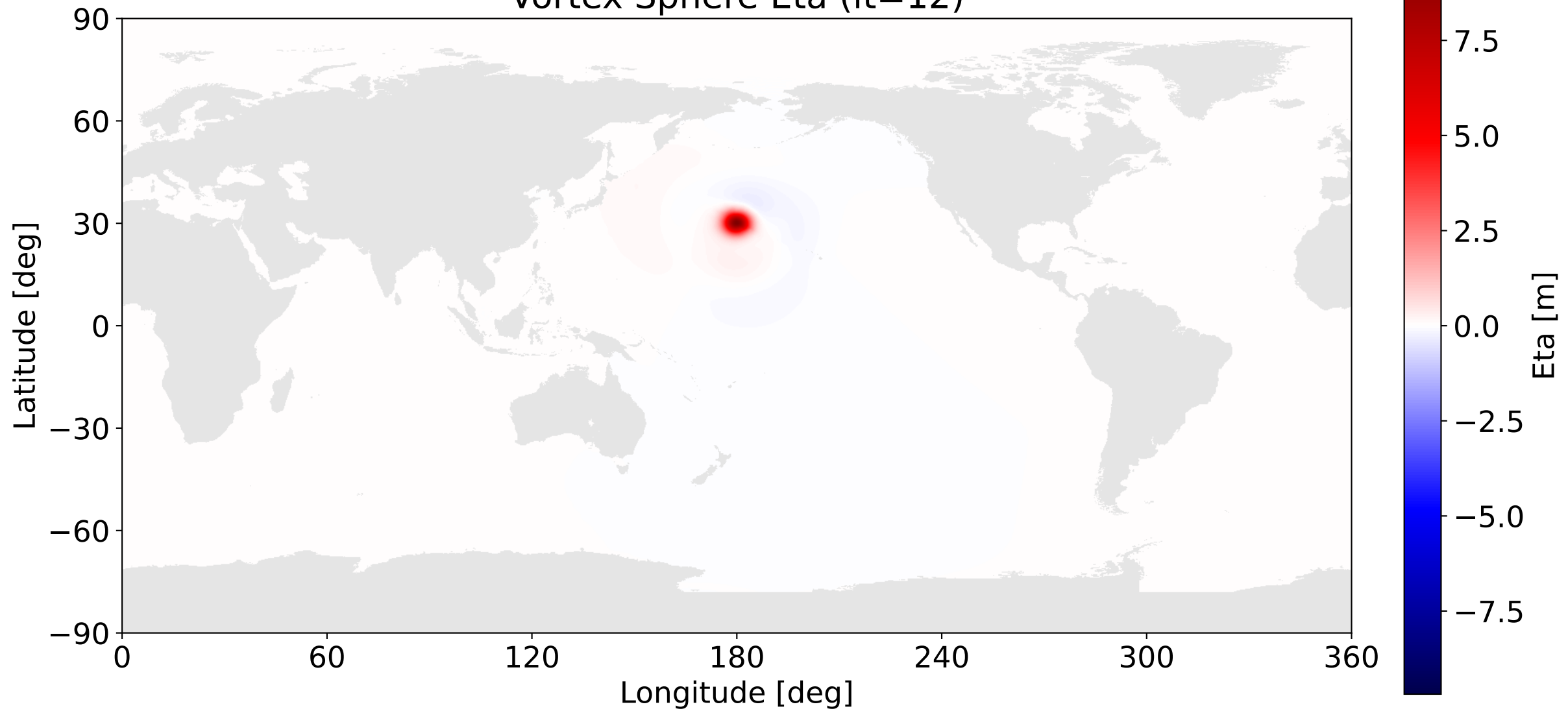
Vortex Sphere Eta (it=12)
