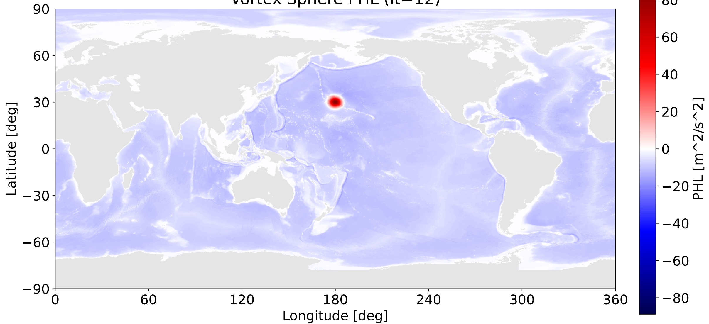
Vortex Sphere PHL (it=12)
