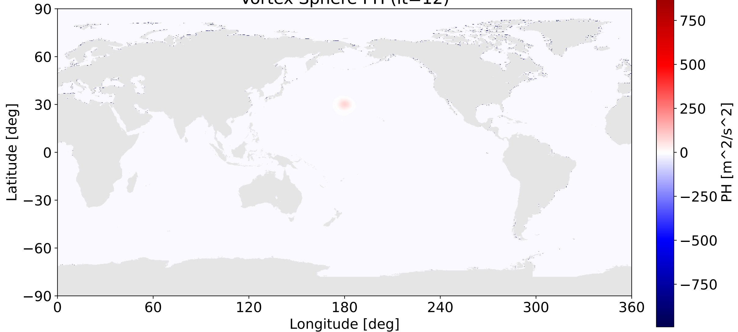
Vortex Sphere PH (it=12)
