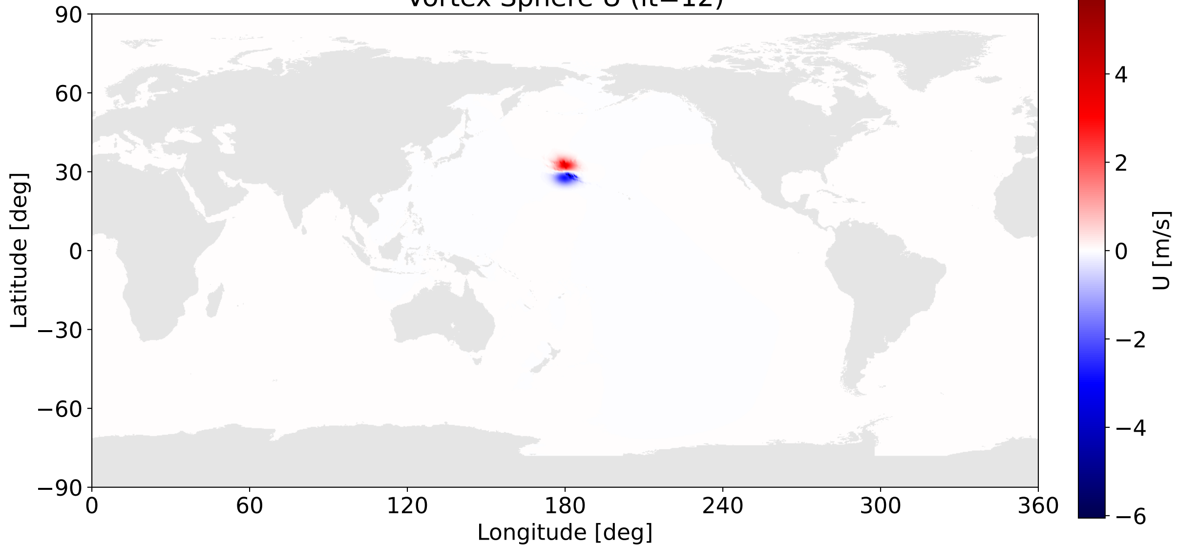
Vortex Sphere U (it=12)
