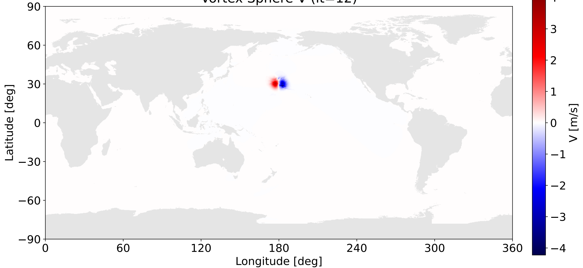
Vortex Sphere V (it=12)
