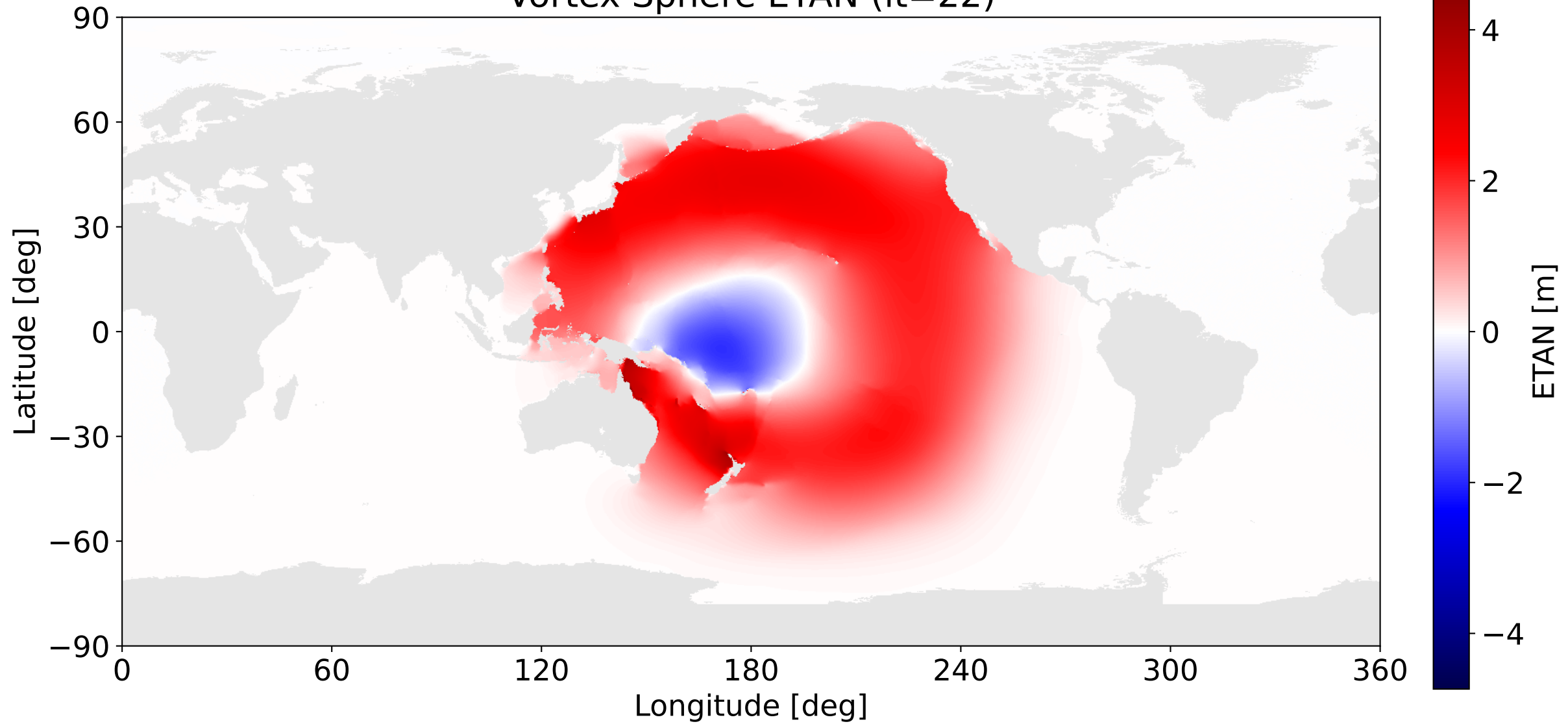
Vortex Sphere ETAN (it=22)
