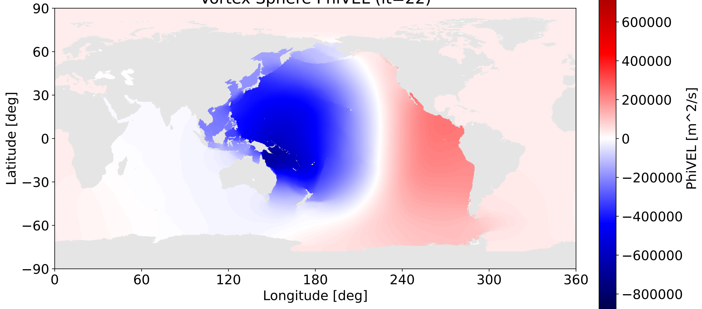
Vortex Sphere PhiVEL (it=22)
