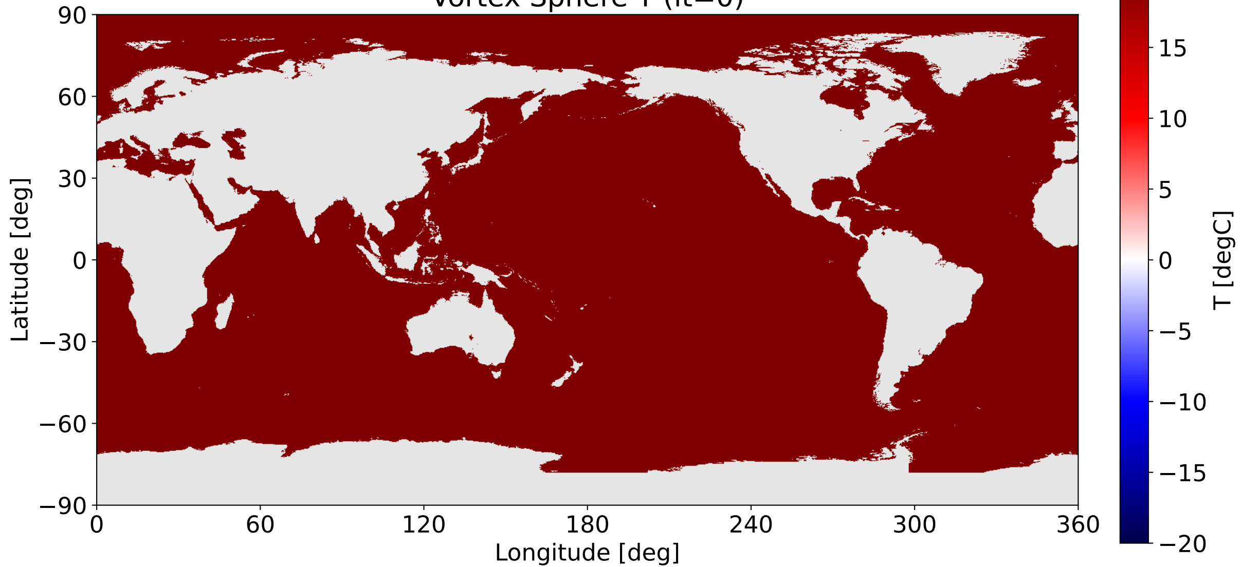
Vortex Sphere T (it=0)
