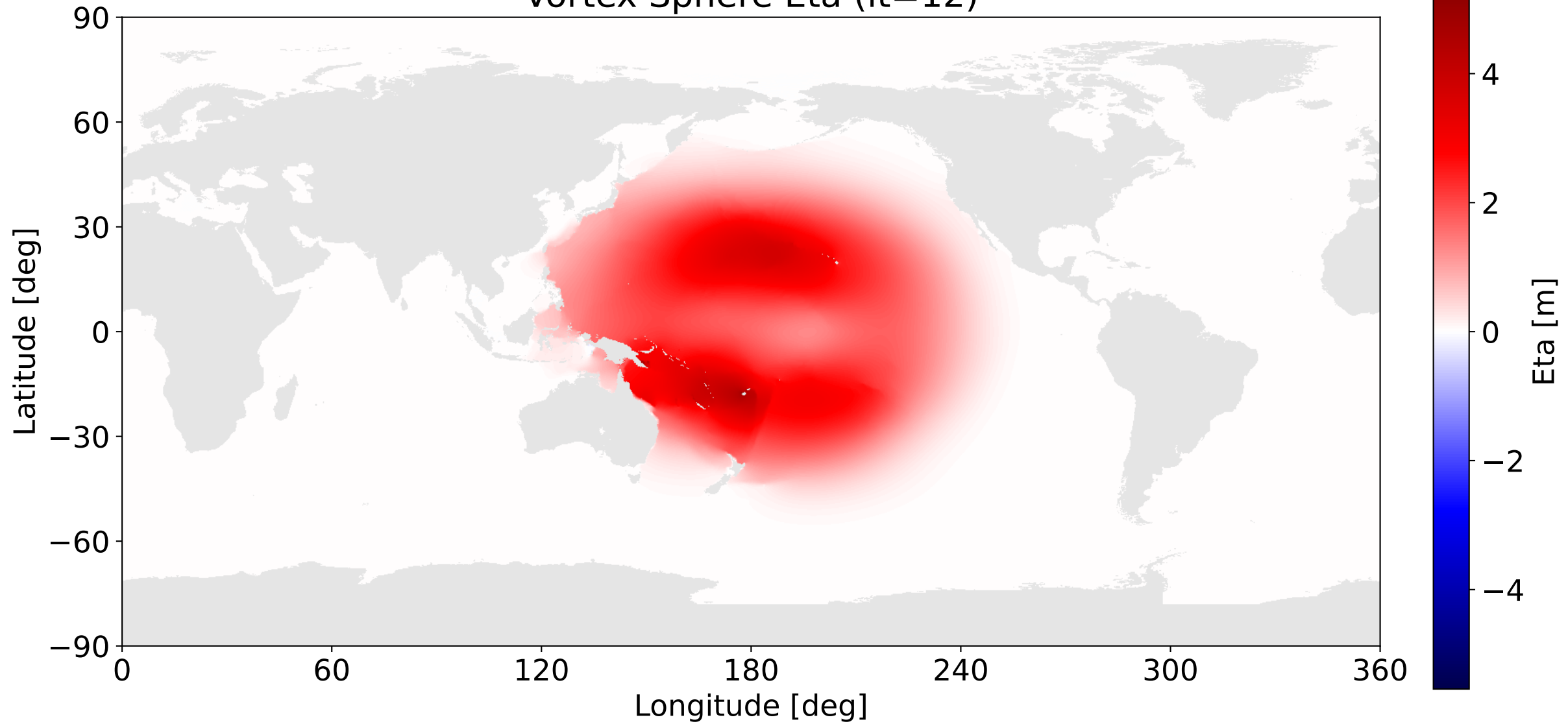
Vortex Sphere Eta (it=12)
