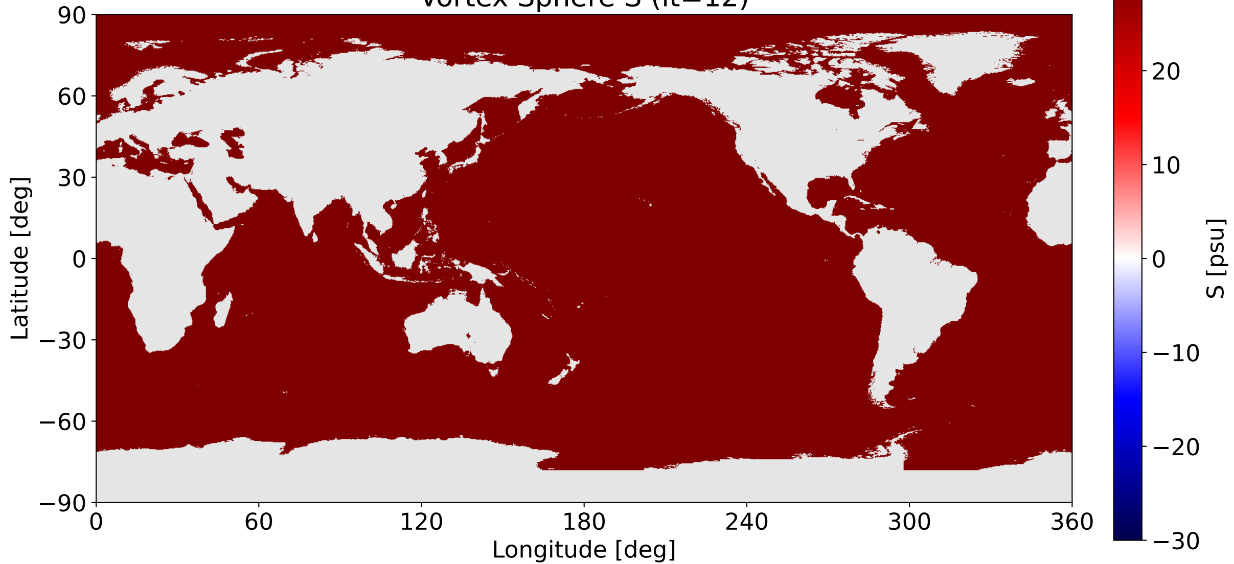
Vortex Sphere S (it=12)
