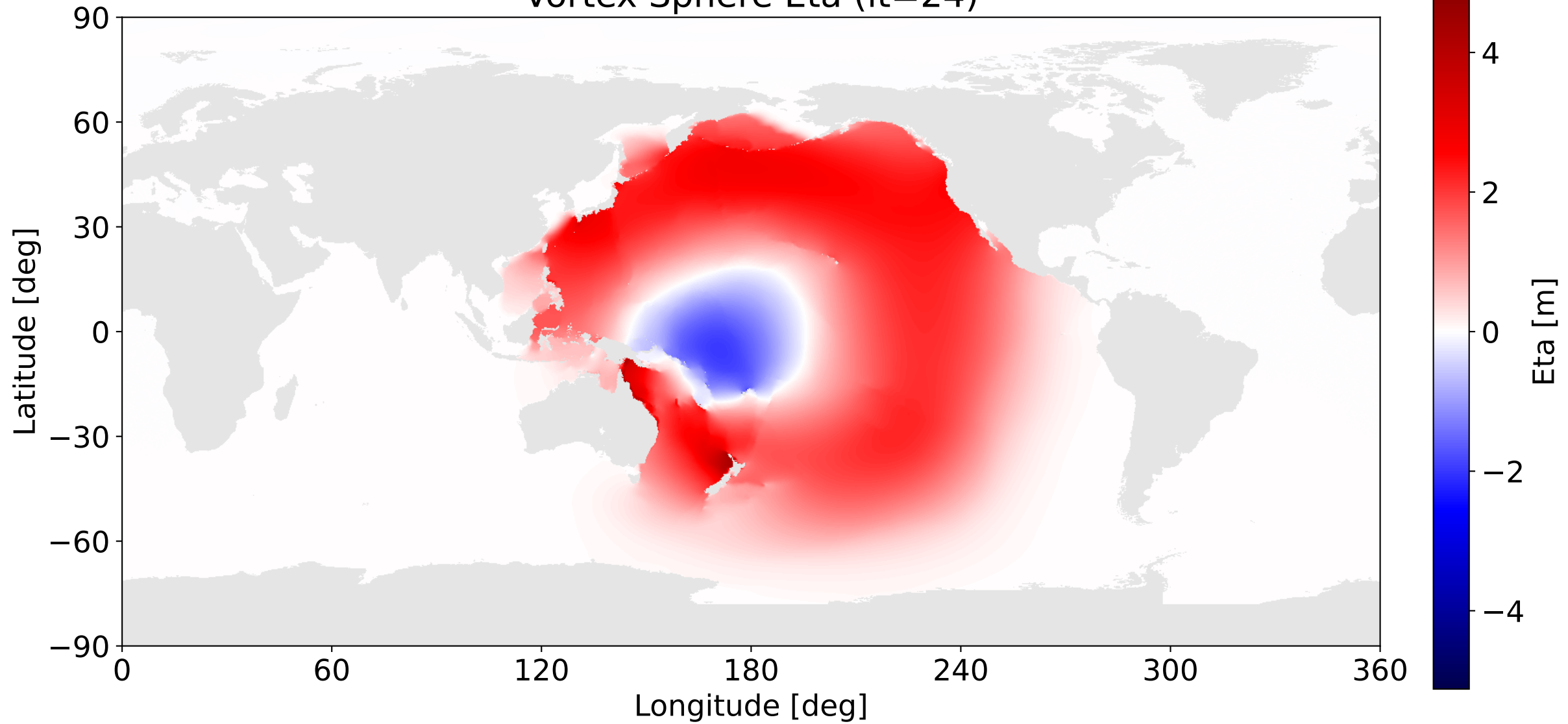
Vortex Sphere Eta (it=24)
