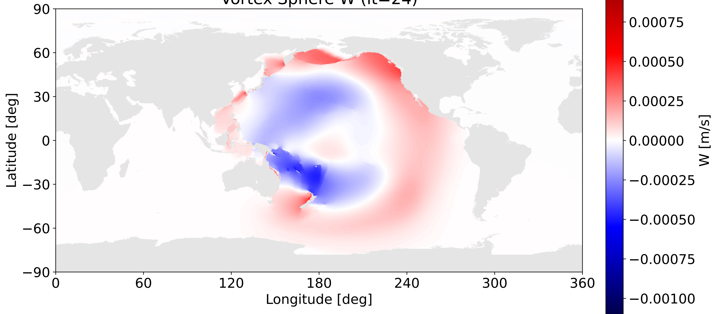
Vortex Sphere W (it=24)
