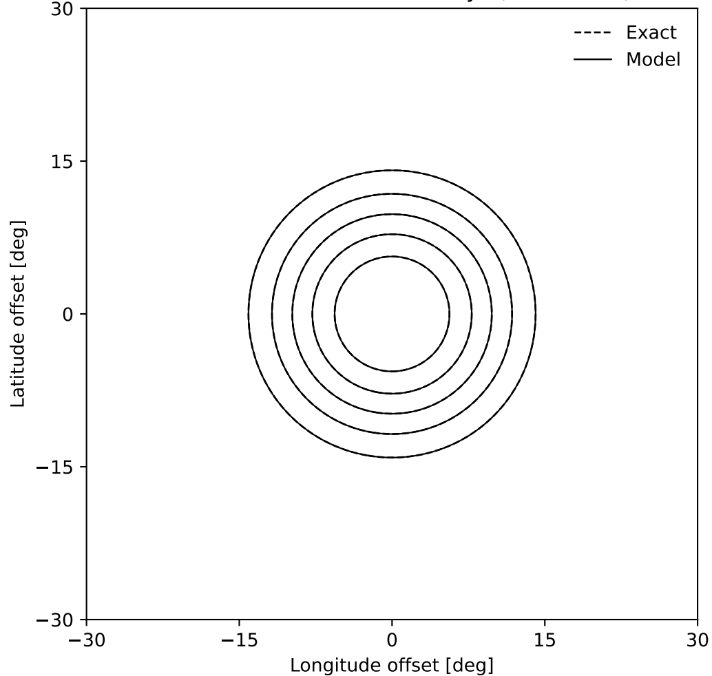
Eta contours at t = 12.00 days (it = 17280)
