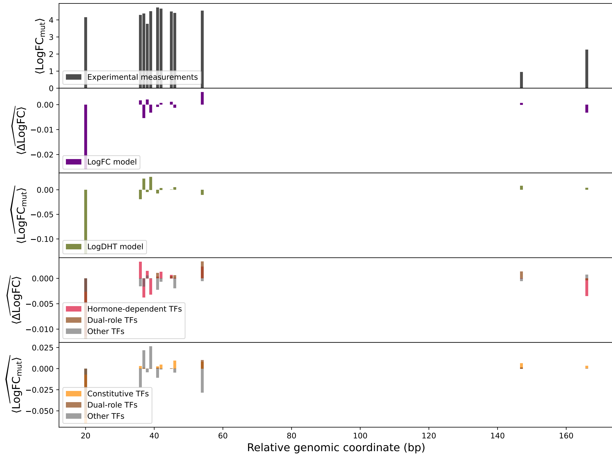
peakno_1185
