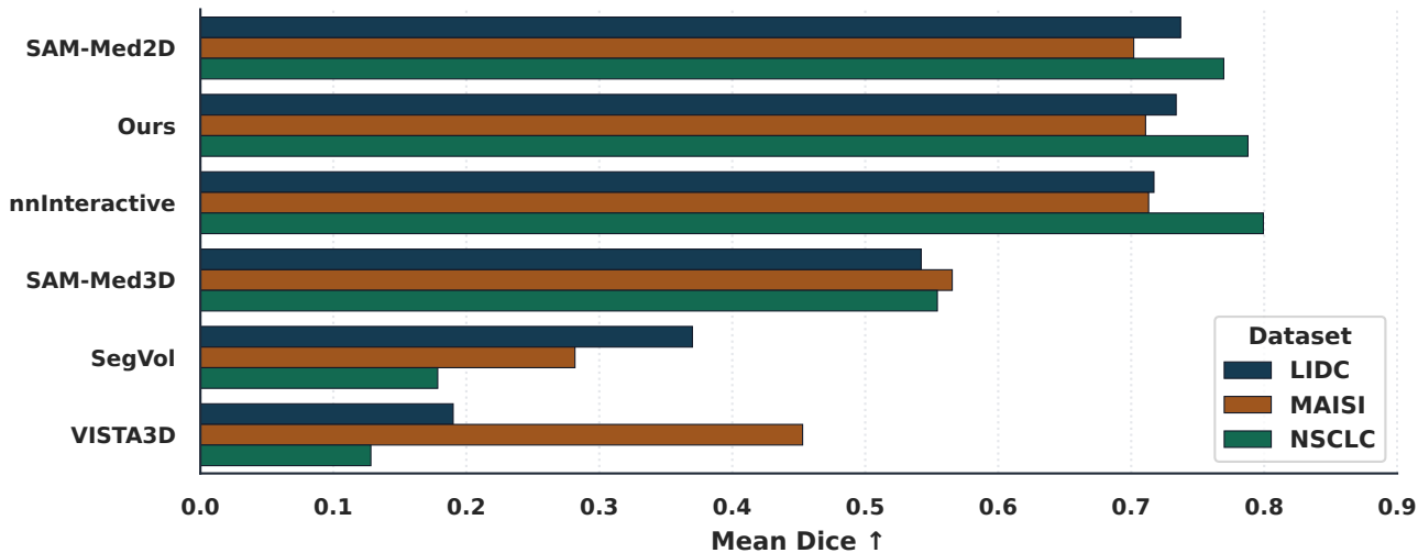
Matched box prompts · LIDC / MAISI / NSCLC
