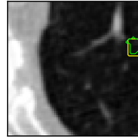
SegVol
