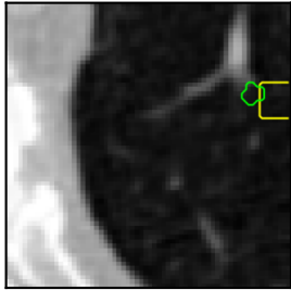
SAM-Med2D
