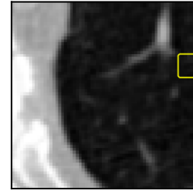
VISTA3D
