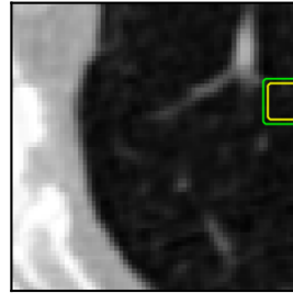
SAM-Med3D
