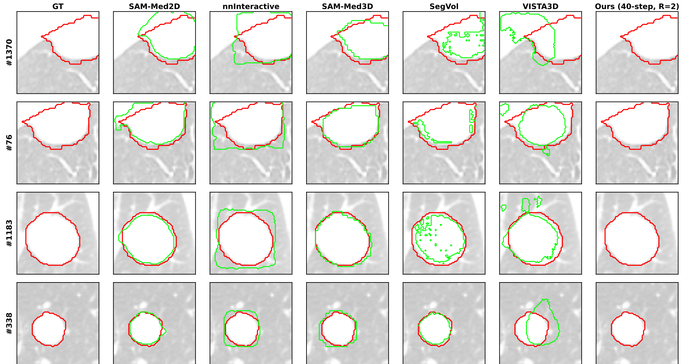
LIDC — red=GT, lime=prediction
