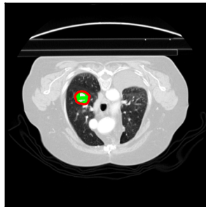
SAM-Med2D
