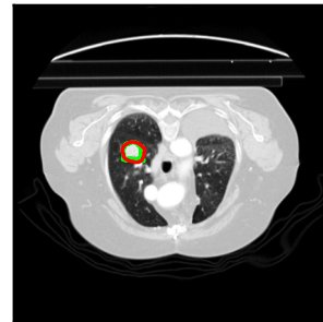
SAM-Med3D
