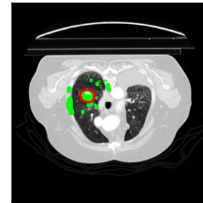
VISTA3D
