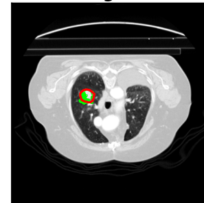
SegVol
