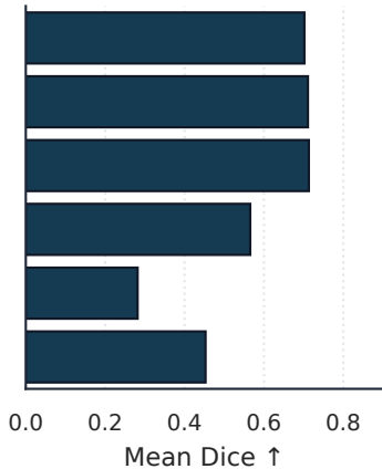
dataset = MAISI
