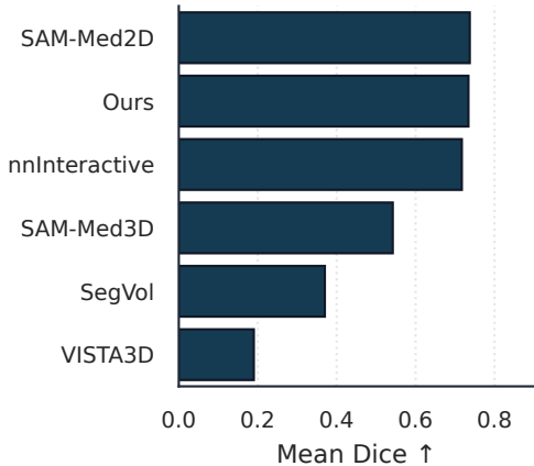
dataset = LIDC
