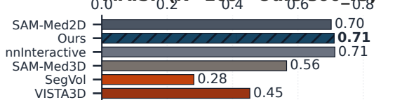
NSCLC (N=85 · Ours s60_r1)
