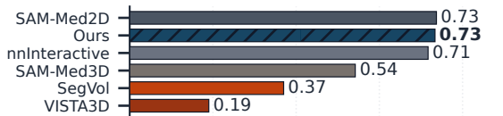
MAISI (N=109 · Ours s60_r3)
