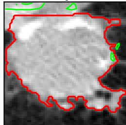
40-step, R=2
