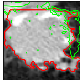
80-step, R=2
