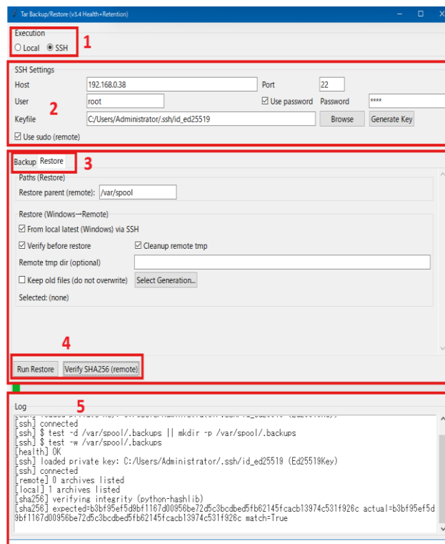
図 2 : TB SafeBox メイン画面の構成
