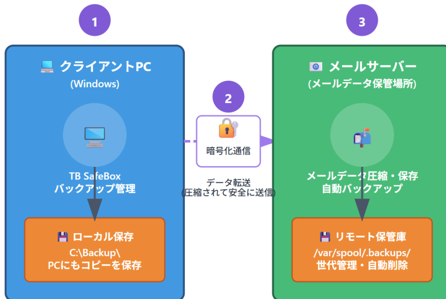
図 1：バックアップ処理の流れ
