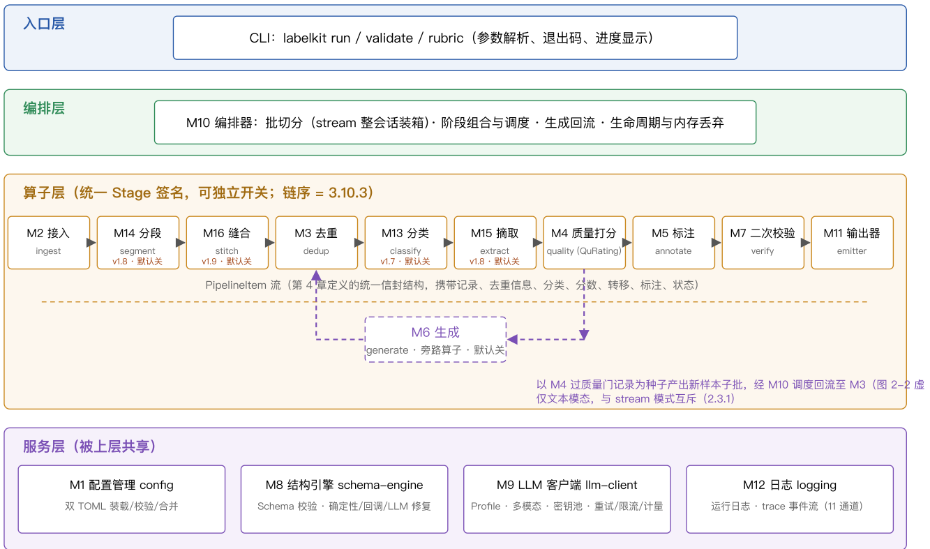
图 2-1 LabelKit 总体架构（四层）。实线为算子层主链数据流；紫色虚线为 M6 生成的旁路（取种子 / 子批回流，v1.3 拆分为独立模块）。v1.7 算子层增 M13 classify（3.13，主链工位任 M3 与 M4 之间）。v1.8 算子层增 M14 segment 与 M15 extract（3.14、3.15，默认关）：M14 工位在主链最前（M3 之前，消费 M2 会话流视图产出 episode），M15 工位任 M13 与 M4 之间（对序列信封写入转移）。v1.9 算子层增 M16 stitch（3.16，默认关）：工位任 M14 与 M3 之间（把会话内碎片缝合为线索——缝合改成员集，先于判重与摘取）。
