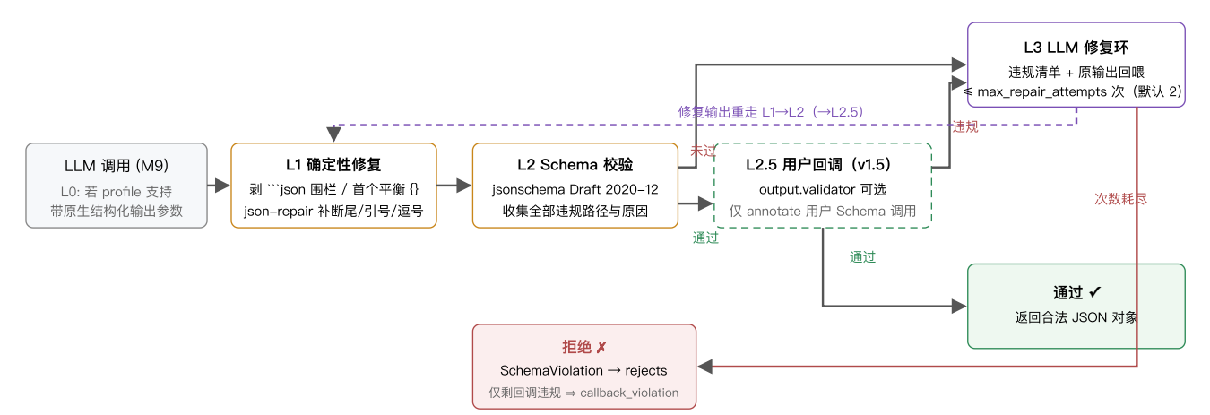
图 3-3 结构引擎四层保证。任何写入主输出的对象必然经过 L2 通过分支。
