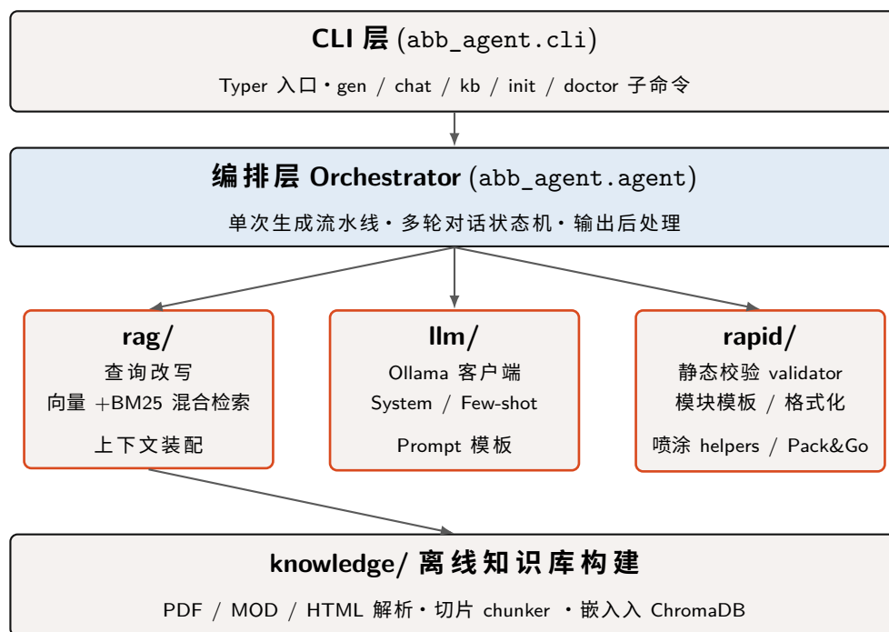
图 1. abb-offline-coder 四层架构（CLI / 编排 / 能力 / 知识库）
