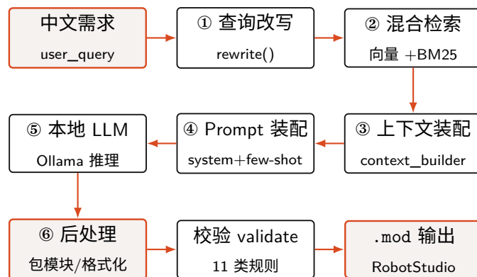
图 2. 单次生成的六级流水线 (query rewrite → retrieve → assemble → prompt → LLM → post-process)
