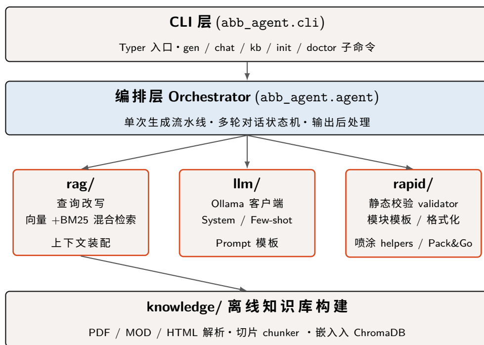
图 1. abb-offline-coder 四层架构 (CLI / 编排 / 能力 / 知识库)
