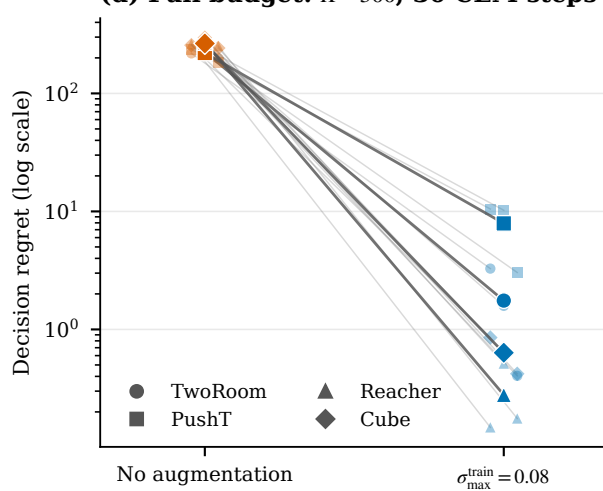
(d) Full budget: K=300 , 30 CEM steps
