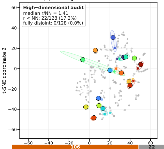
(a) No augmentation · Encoder
