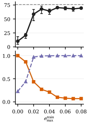
(b) PushT
