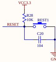
RESET复位
