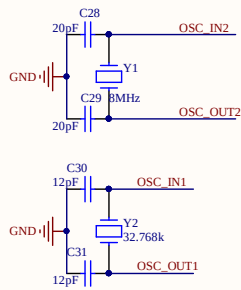
系统时钟晶振
