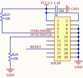
JTAG调试接口
