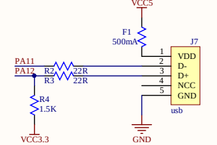
USB 5V供电
