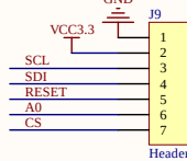
OLED液晶接口
