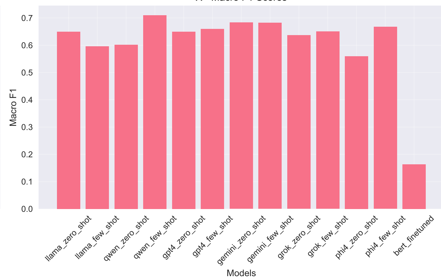
Meeting_Minutes - Macro F1 Scores
