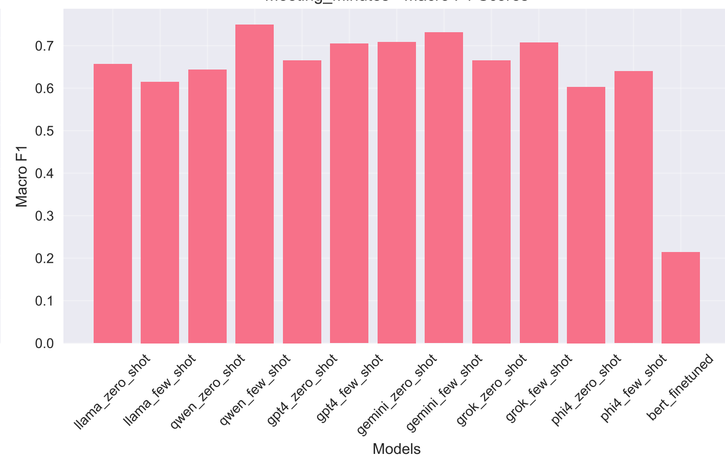
Meeting_Minutes - Macro F1 Scores
