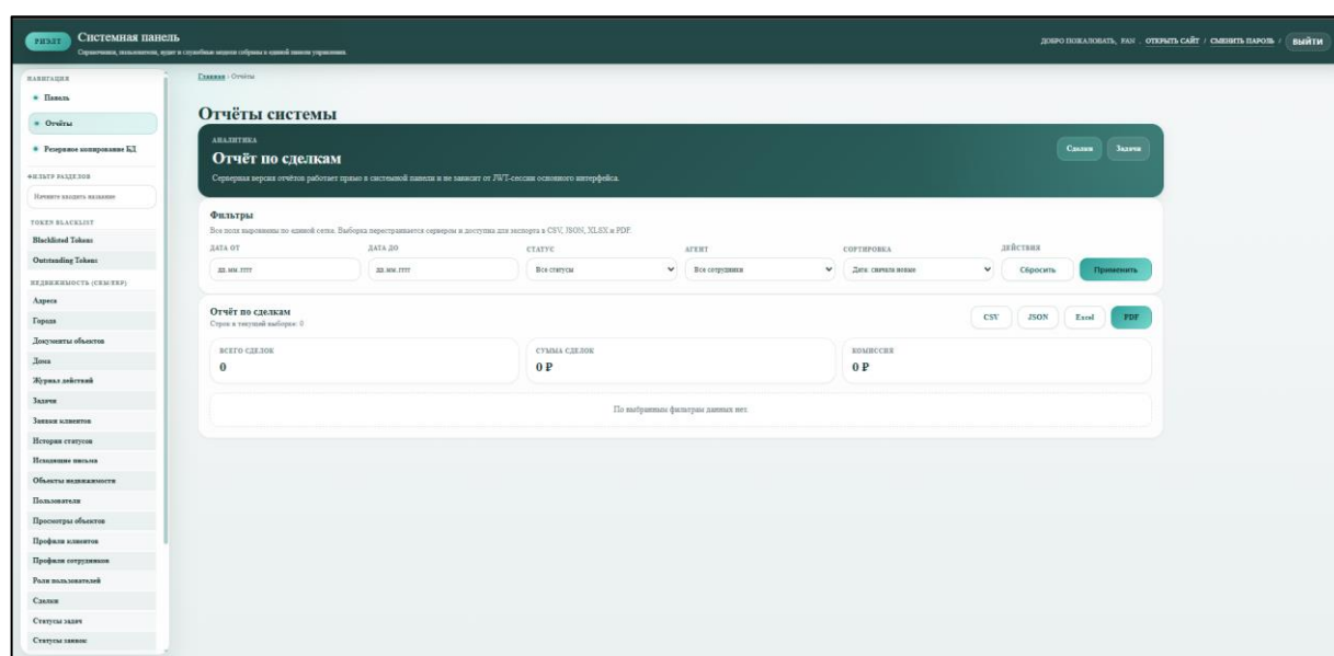
Рисунок 21 – Страница отчёта
