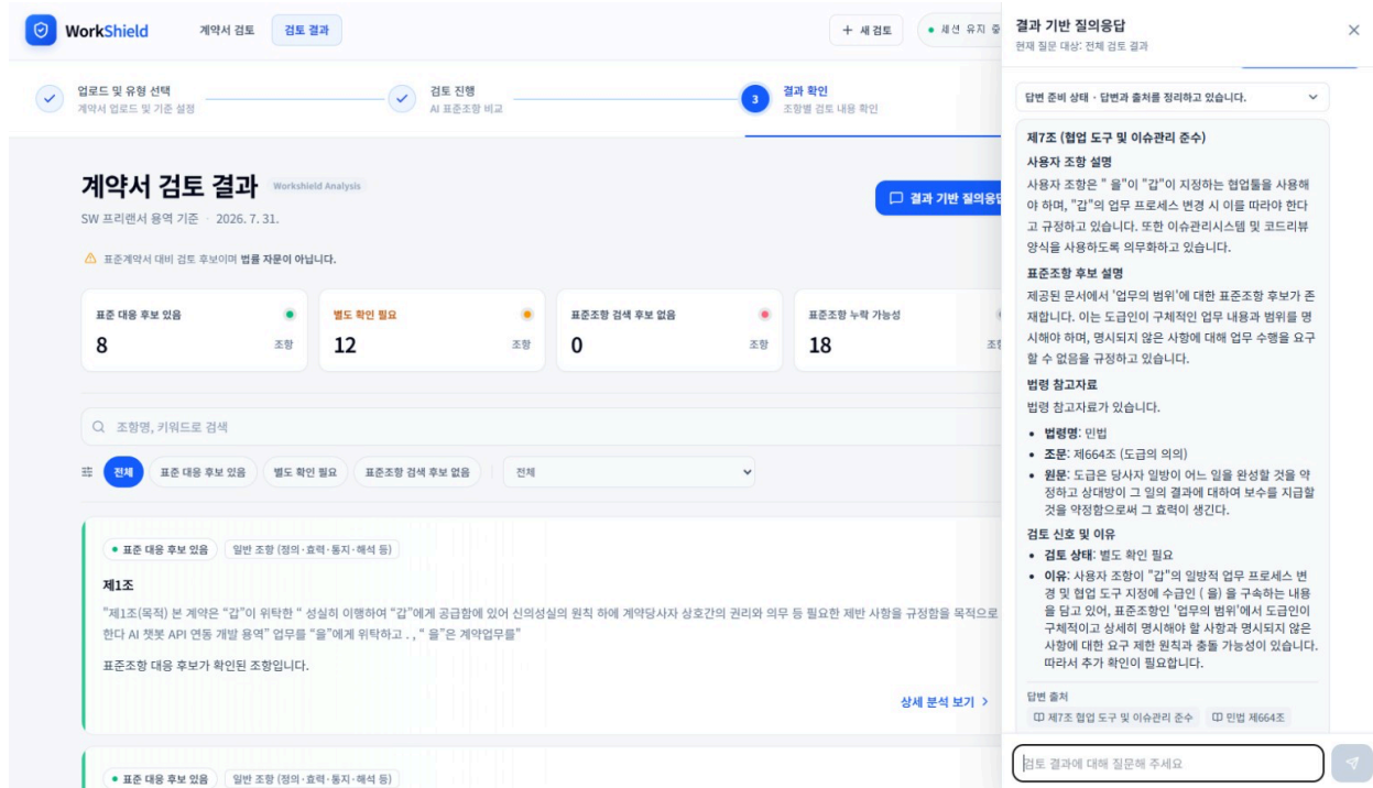
그림 1. WorkShield 계약서 검토 결과 및 결과 기반 질의응답 화면
