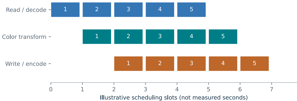
图 8 三阶段流水线的概念时序。颜色阶段始终按块顺序提交，读取与写入可与相邻块重叠。图中时间段是教学示意，不是从性能日志提取的实际甘特图。
