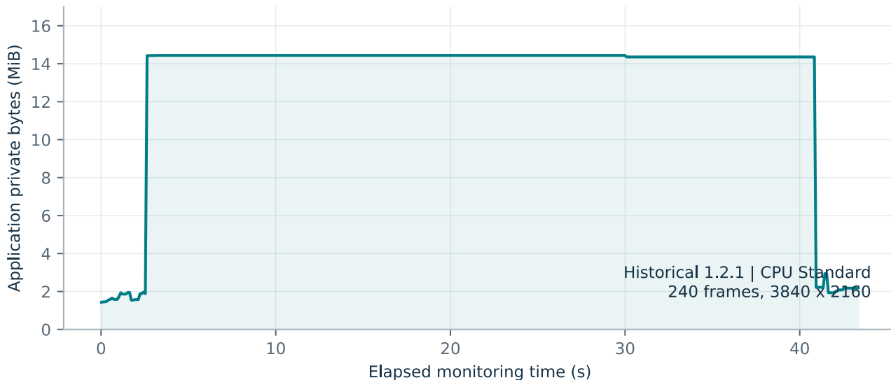
图 16 历史 1.2.1 论文复测的 240 帧 4K120 CPU 标准模式应用私有内存曲线。数据来自 sustained-report.json；仅计主应用，不包含 FFmpeg 子进程或 GPU 显存。曲线是一次运行观察。
