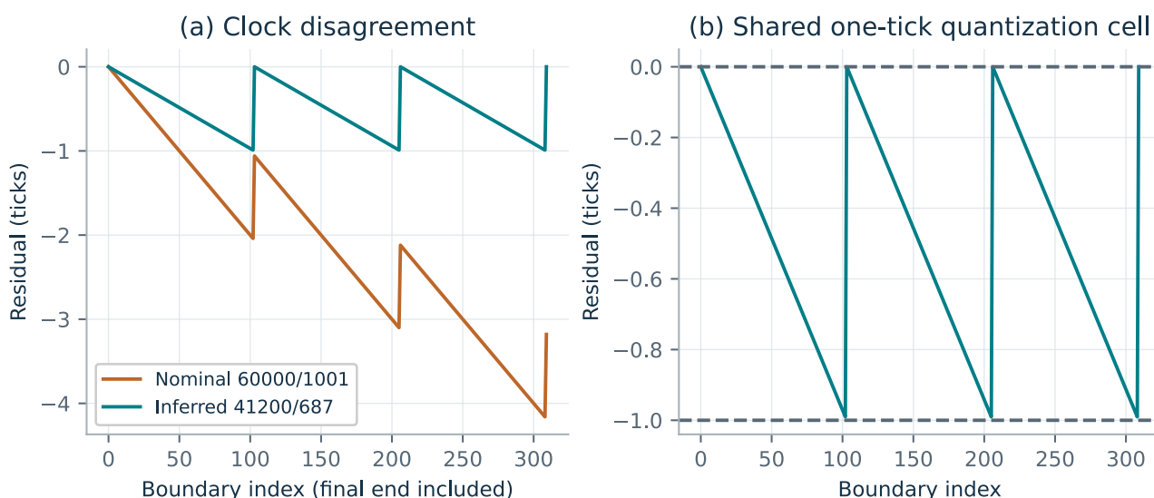
图 10 1.3.0 的 309 包生成重构。左图比较名义与推断时钟残差；右图展示全部边界的共同 tick 单元，含最终包结束。
