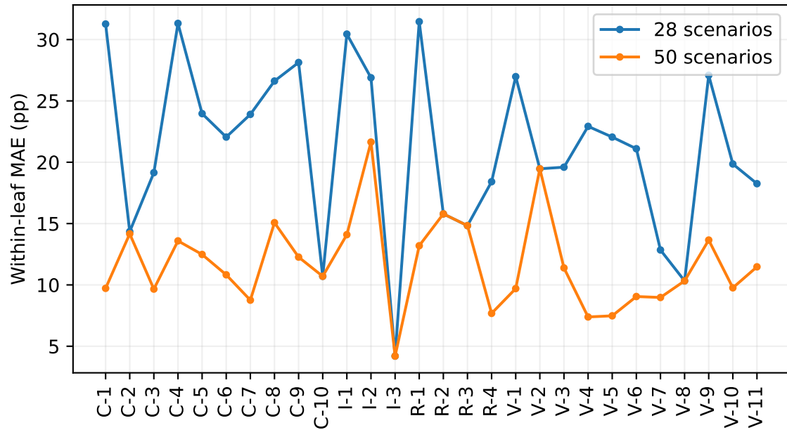
DS
