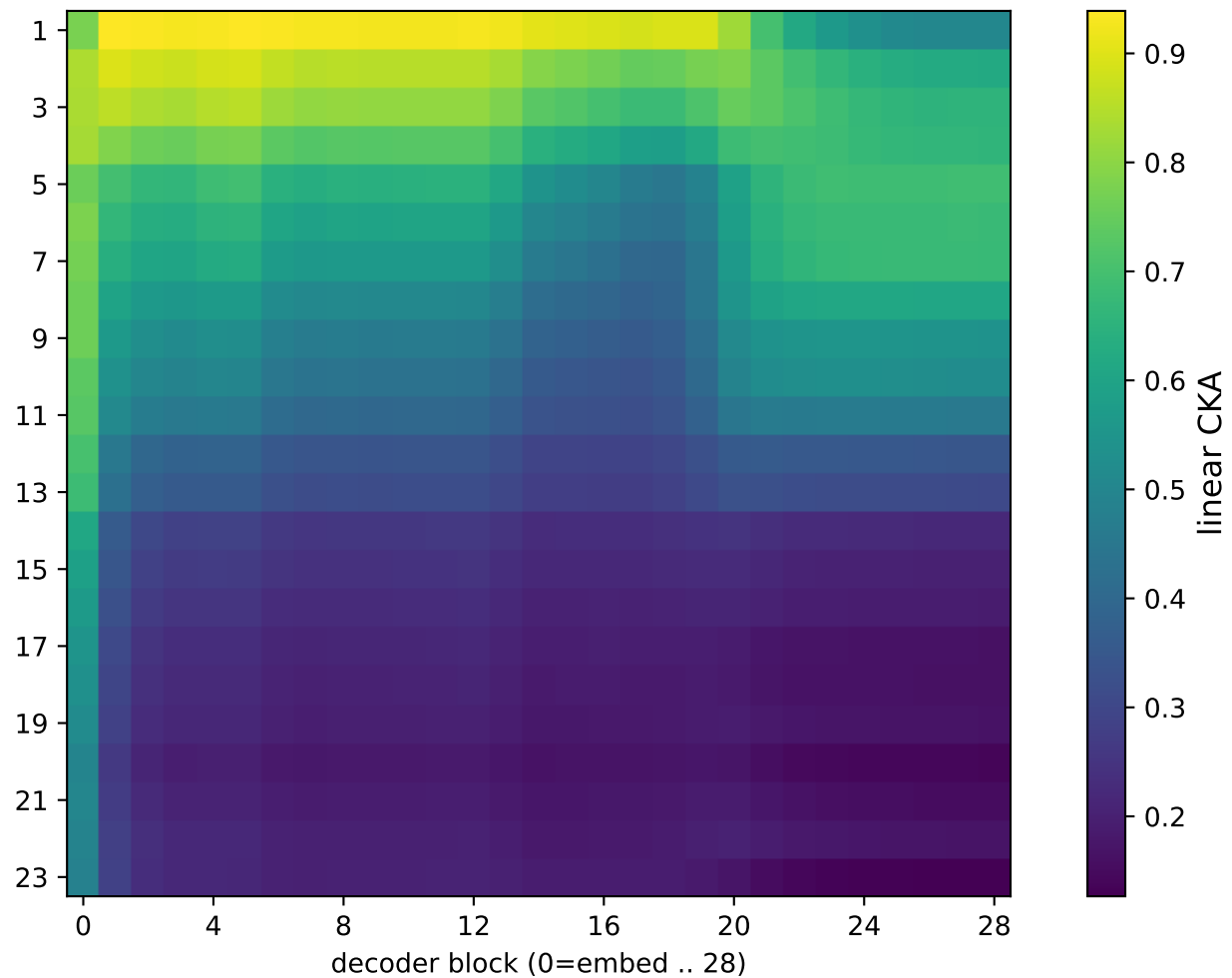
RAEv2 K=23
