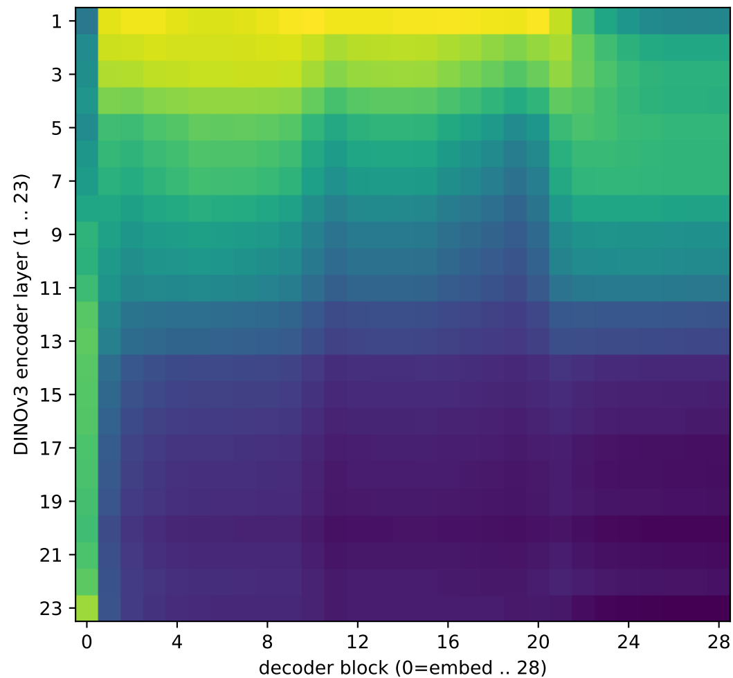
OmniRAE (ours)
