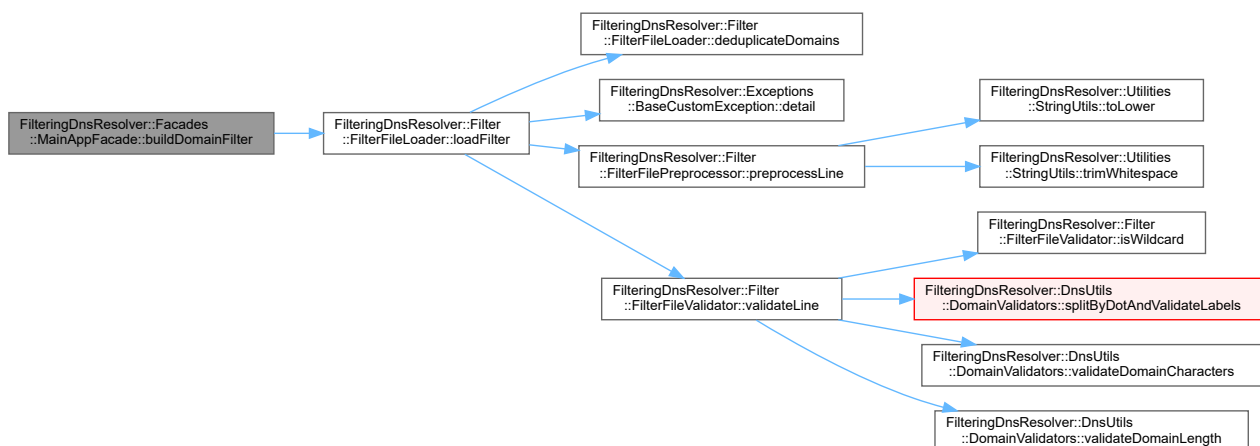
Obrázek 15: Call graph třídy Facades::MainAppFacade
