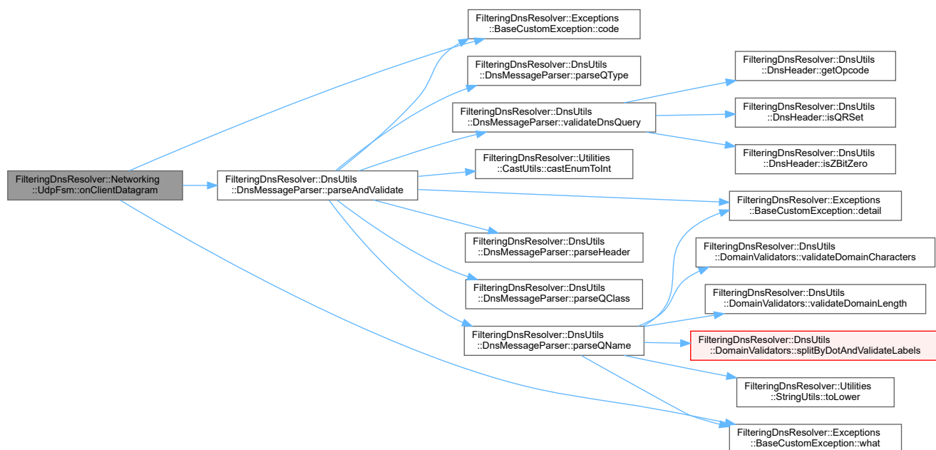
Obrázek 15: Call graph v rámci metody Networking::UdpFsm::onClientDatagram()
