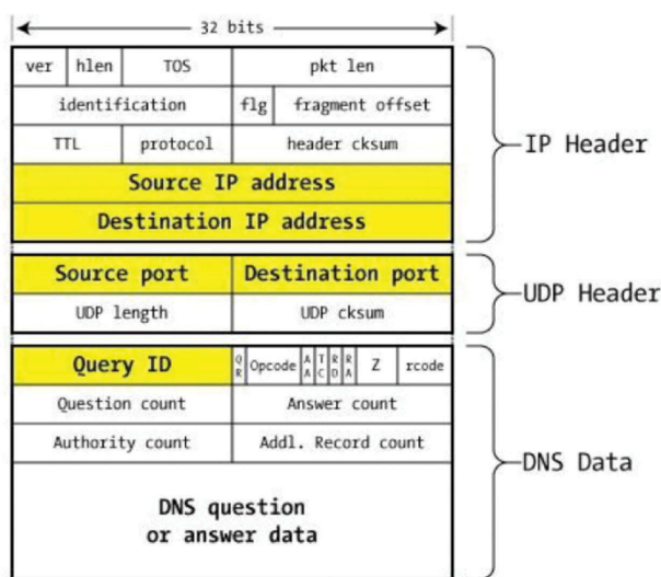
Obrázek 1: Struktura DNS paketu [21]
