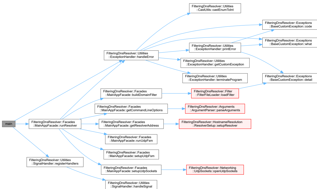
Obrázek 2: Graf volání z funkce main()
