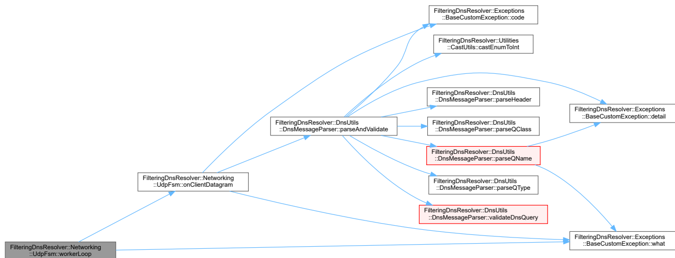
Obrázek 14: Call graph v rámci pracovních vláken Networking::UdpFsm::WorkerLoop()
