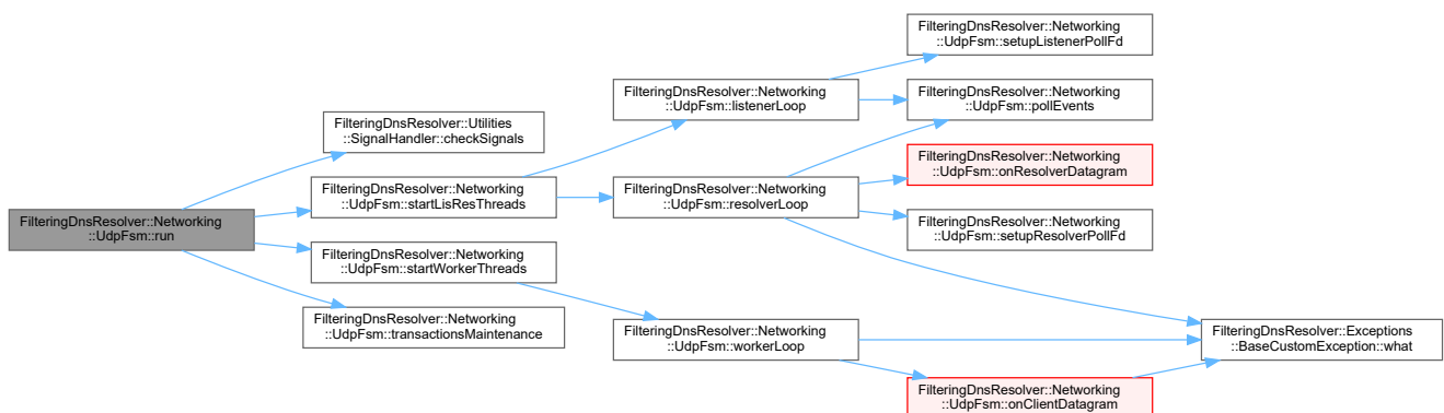
Obrázek 13: Call graph třídy Networking::UdpFsm
