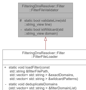
Obrázek 11: Třída Filter::FilterFileValidator
