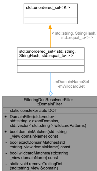
Obrázek 10: Třída Filter::DomainFilter
