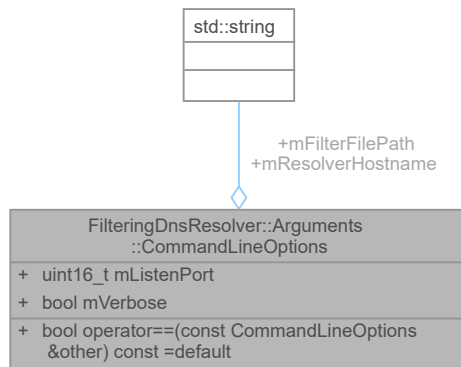
Obrázek 3: Obsah datové třídy Arguments::CommandLineOptions
