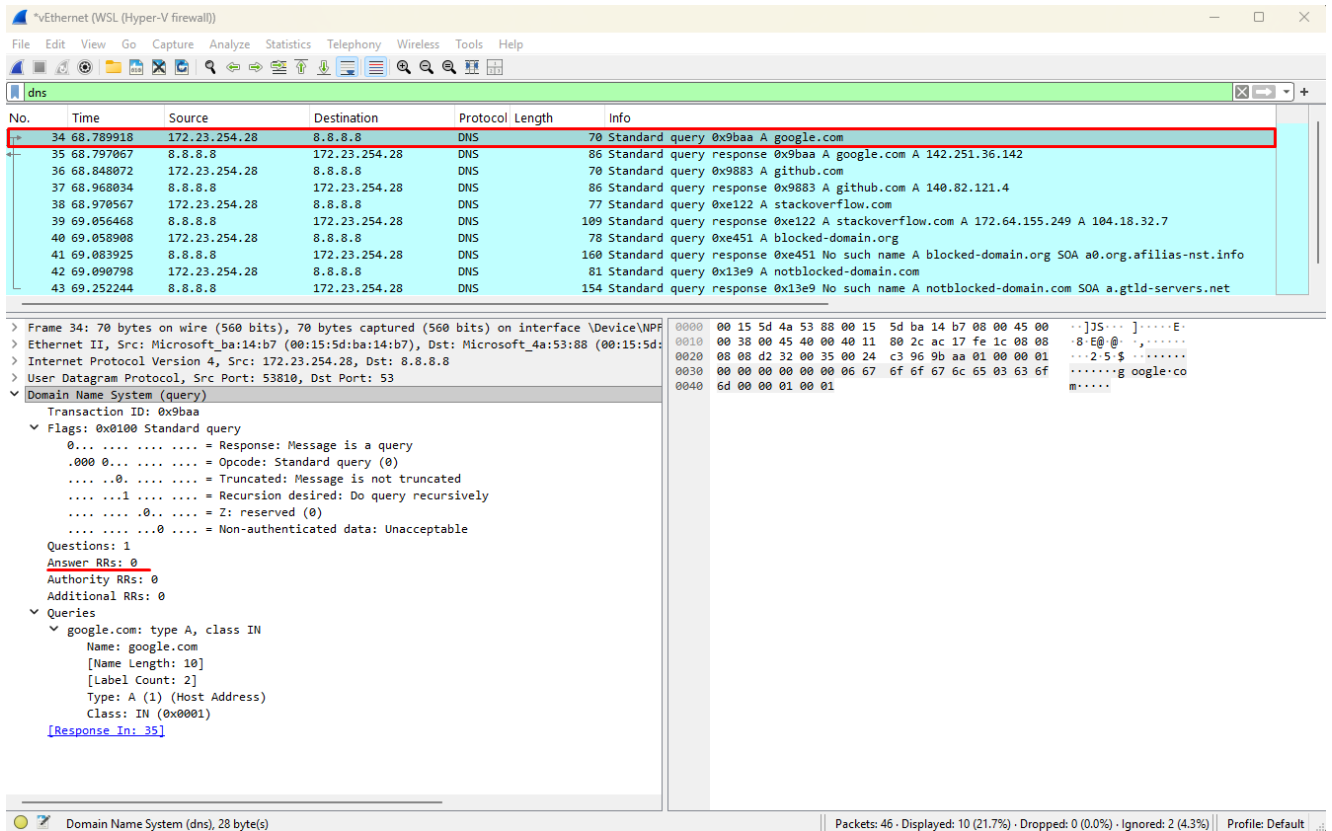
Obrázek 17: Ukázka forwardování povolených domén – forwarding dotazu na upstream resolver`
