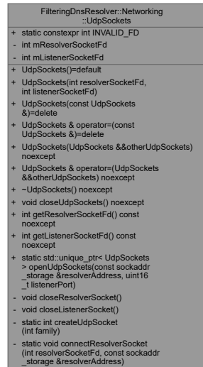
Obrázek 12: Třída Networking::UdpSockets
