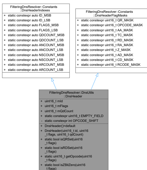
Obrázek 4: Třída DnsUtils::DnsHeader
