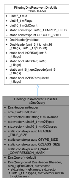
Obrázek 5: Třída DnsUtils::DnsQuery
