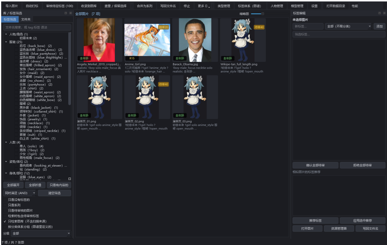
图 4-1 主界面全貌
