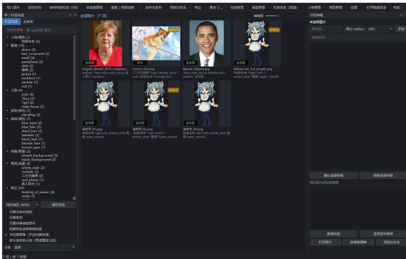
图 4-1 主界面全貌
