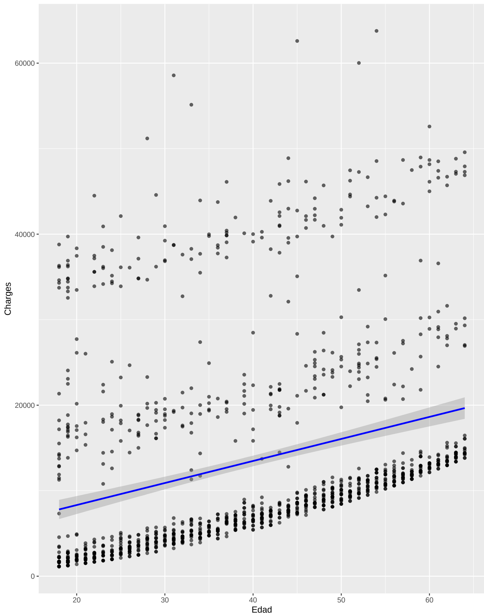
Gráfico de Dispersión: Charges vs Age
